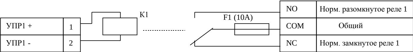
схема подключения УУК-12-01/1, УУК-24-01/1
