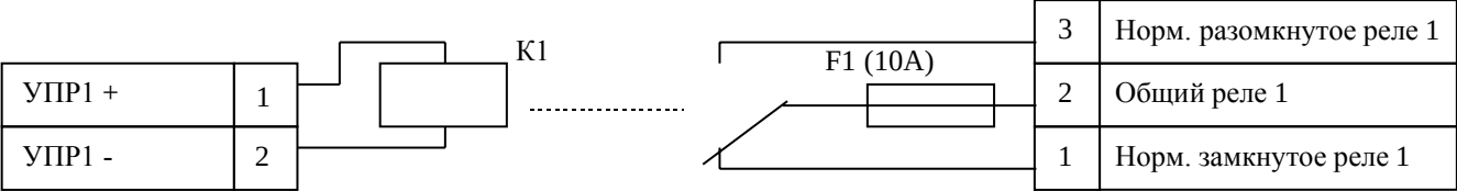
схема подключения УУК-12-02, УУК-24-02, УУК-12-02 уличный, УУК-24-02 уличный
