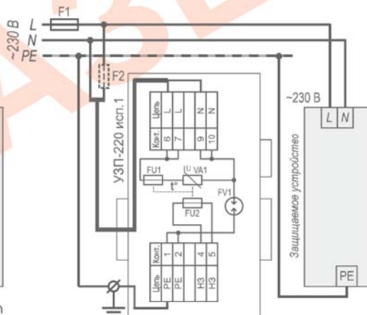
Рисунок 3 – Схема подключения устройства более 16 А
