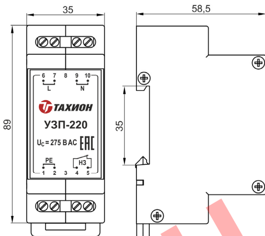
Рисунок 1 – Габаритные и установочные размеры
