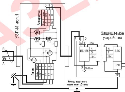
Рисунок 4 – Схема включения 3. Используется в трехпроводных системах связи, в которых для устранения влияния разности потенциалов между сигнальными землями (SG) устройств применяются приемно-передатчики с гальванической развязкой.
