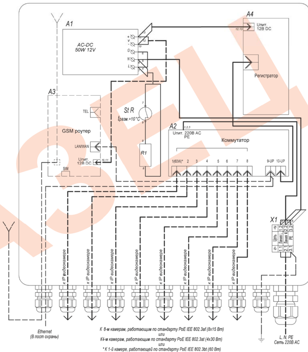
Рис.2 Схема электрическая принципиальная
