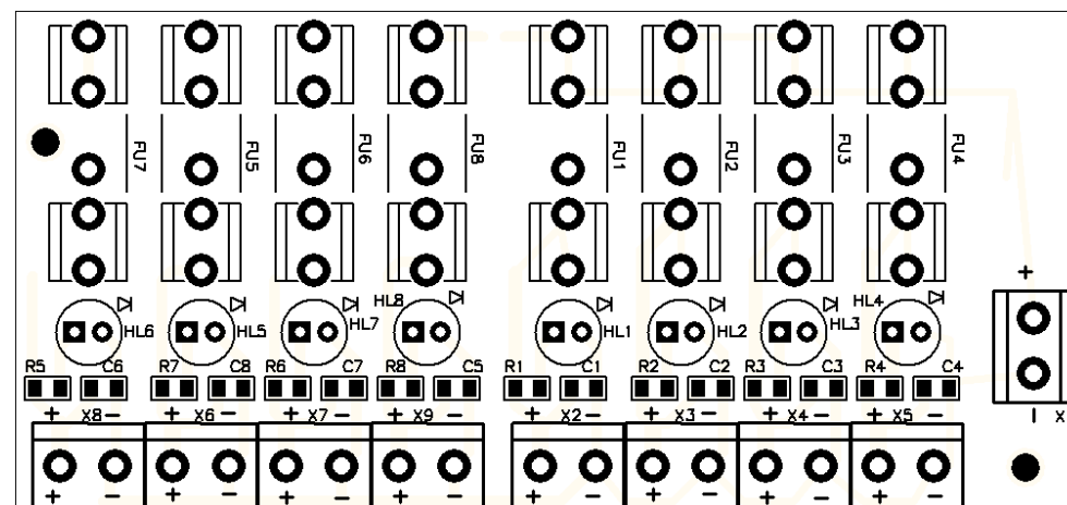
Рис. 1. Схема подключения УЗК-8
