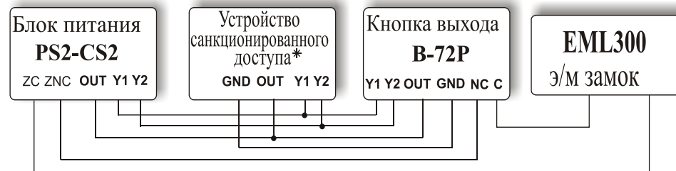
Схема подключения В-72Р в составе домофонного комплекса ELTIS5000.
