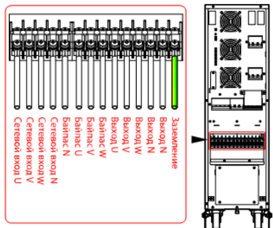
Рис. 3-13 Схема подключения для режима 3/3
