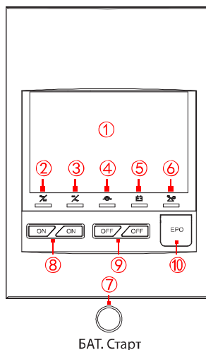
Рис. 2-5 Панель управления
