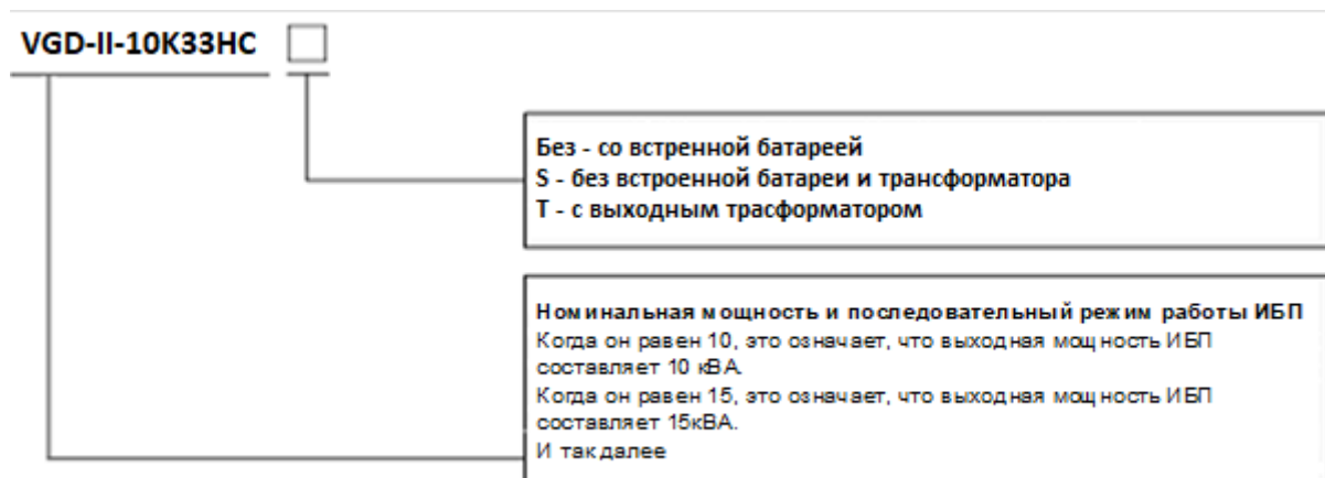
Рис. 2-1 Описание модели
