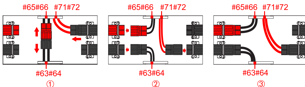
Рис. 3-23 Схема подключения коннекторов для режима 3/1
