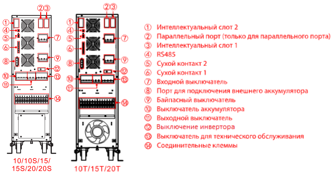
Рис. 2-6 Вид задней панели VGD-II-10-20K33HC
