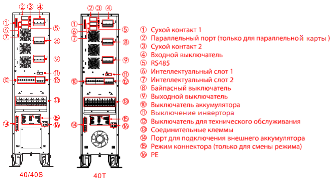
Рис. 2-8 Конструкция задней панели VGD-II-40K33HC
