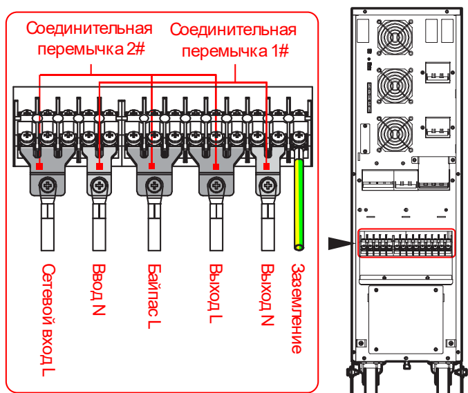
Рис. 3-16 Установка соединительных перемычек и схема подключения для режима 1/1
