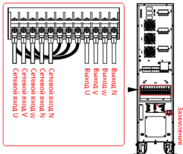
Рис. 3-22 Схема подключения режима 3/3
