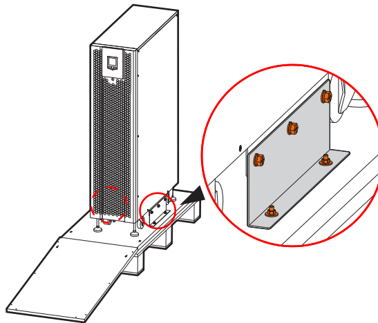
Рис. 3-4 Положение болтов
