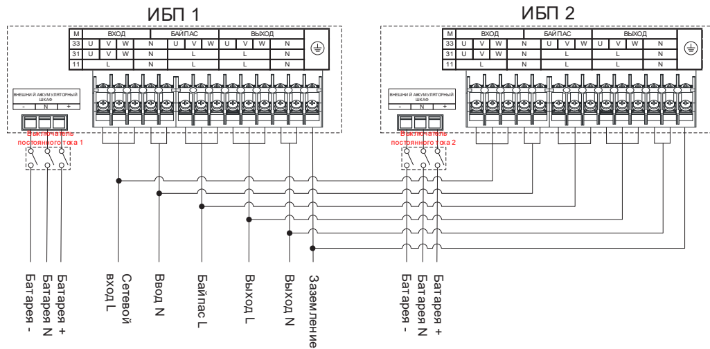
Рис. 3-31 Схема подключения параллельной системы для режима 1/1 VGD-II-10K33HC / VGD-II-10K33HCS / VGD-II-15K33HC / VGD-II-15K33HCS / VGD-II-20K33HC / VGD-II-20K33HCS
