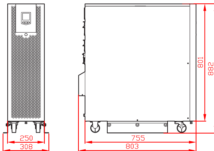
Рис. 3-6 Внешние размеры ИБП VGD-II-10K33HC / VGD-II-10K33HCS / VGD-II-10K33HCT / VGD-II-15K33HCS / VGD-II-15K33HCT / VGD-II-20K33HC / VGD-II-20K33HCT (единица измерения: мм)
