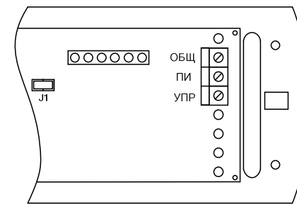
Рис.2. Расположение перемычки J1 на плате изделия.
