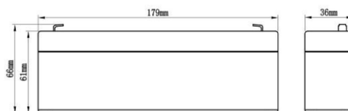
Габаритные размеры, мм
