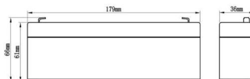
Габаритные размеры, мм
