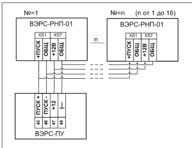
Рис. 7. Схема подключения ВЭРС-РНП-01 к ВЭРС-ПУ.
