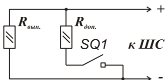
Рис. 5. Схема подключения датчиков с нормально разомкнутыми контактами.
