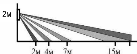
Зона обнаружения в вертикальной плоскости при нормальном режиме чувствительности.
