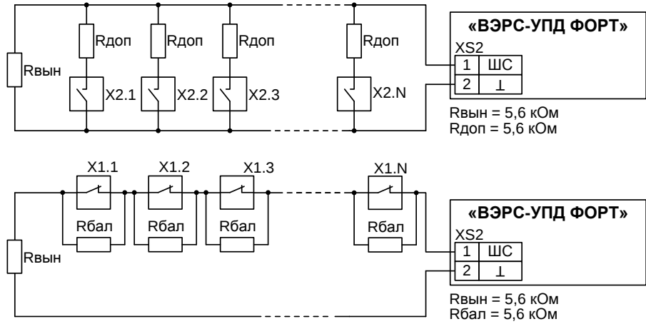
Рисунок 10 Схемы подключения ШС к пожарному типу устройства «ВЭРС УПД-ФОРТ»
