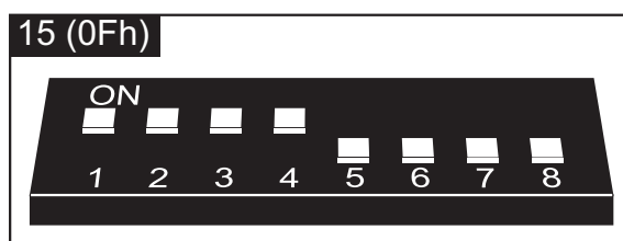
Рис. 20. Способ установки адреса в модуле расширения выходов.
