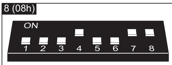
Рис. 15. Способ установки адреса в контроллере ACU-100.
