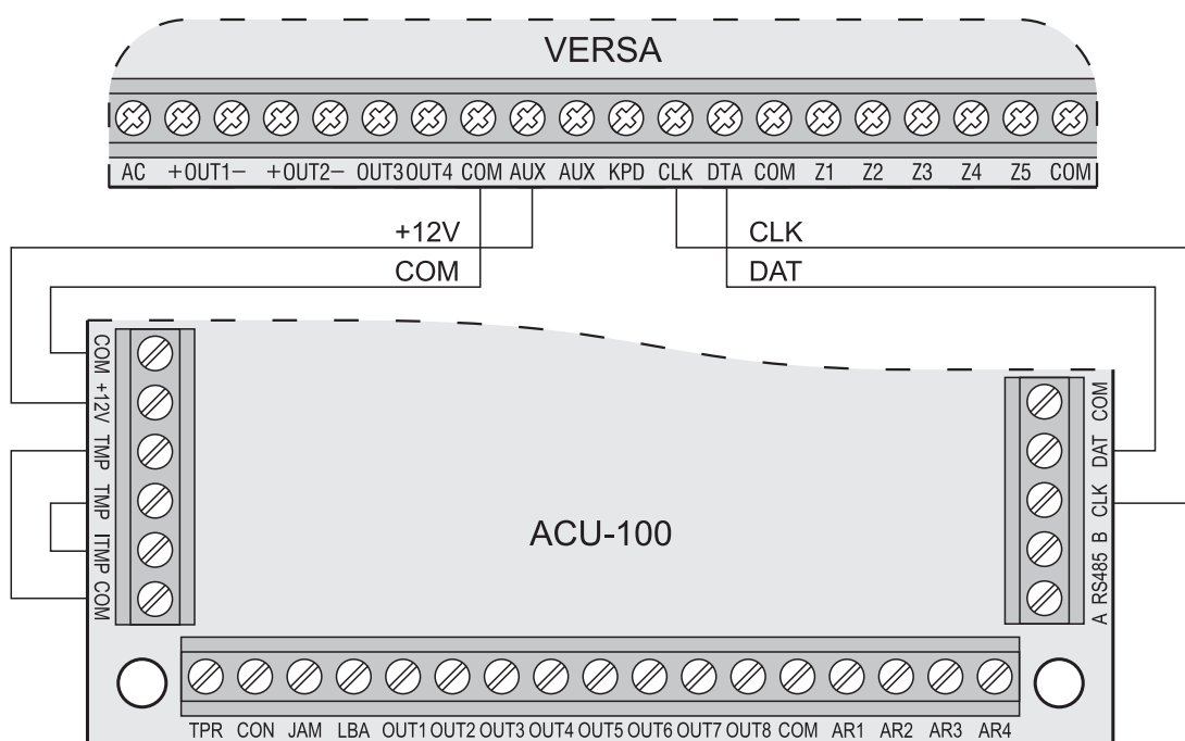
Рис. 16. Способ подключения контроллера ACU-100. Клеммы TMP тамперного контакта контроллера подключены к тамперному шлейфу контроллера (клеммы ITMP и COM), благодаря чему информация о нарушении тамперного контакта контроллера отправляется на ПКП по коммуникационной шине. Если клеммы TMP не подключены к тамперному шлейфу контроллера, клемму ITMP следует замкнуть на массу.
