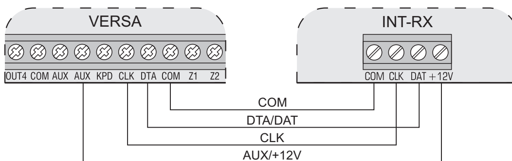
Рис. 14. Способ подключения модуля расширения INT-RX.
