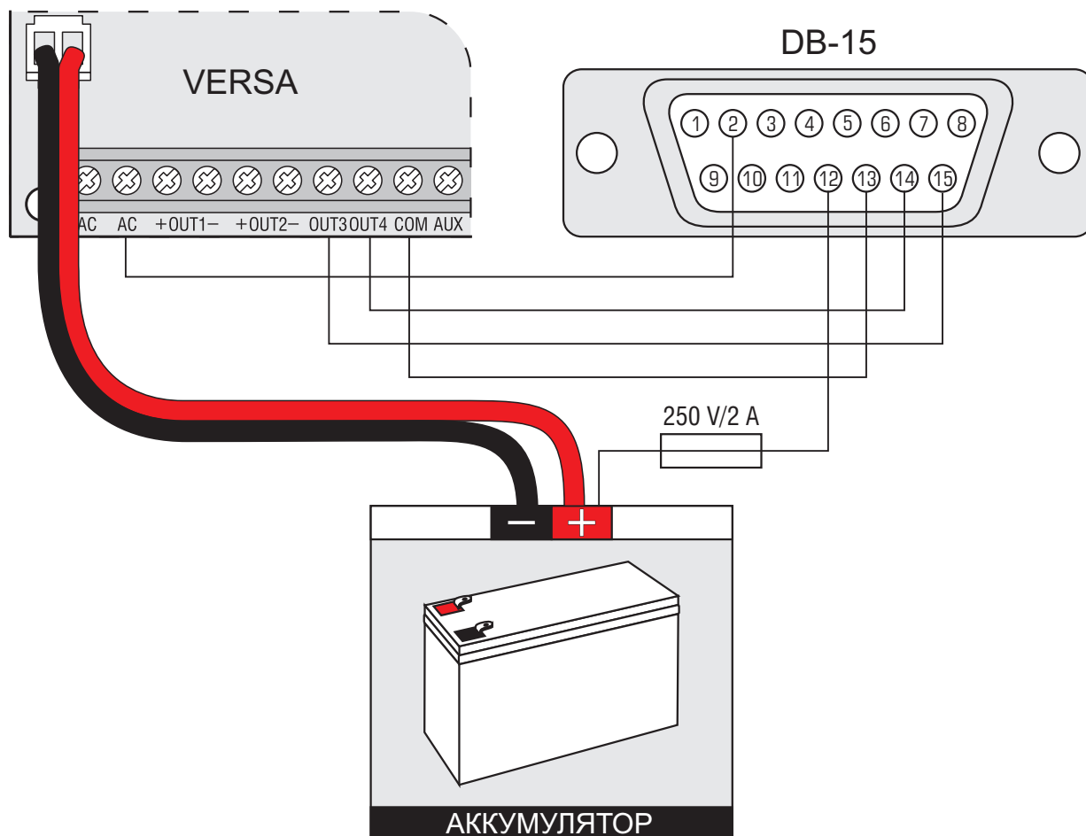
Рис. 29. Способ подключения к ПКП радиопередатчика NR2-DSC фирмы NOKTON. Разъем DB-15 типа «мама» – вид со стороны точек пайки.
