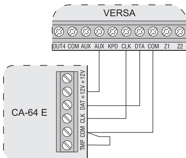
Рис. 18. Способ подключения модуля расширения зон CA-64 E. Модуль расширения установлен в тот самый корпус, как и ПКП, поэтому клемма TMP замкнута на массу COM.
