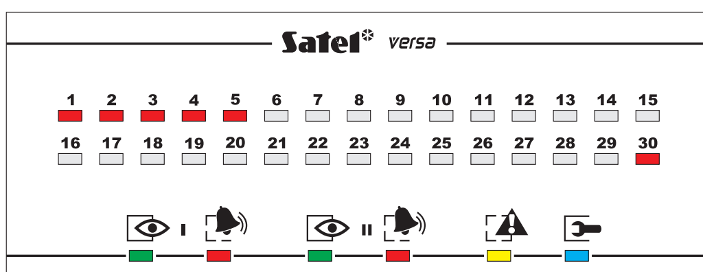
Рис. 9. Программирование адреса светодиодной клавиатуры. Светодиоды с цифрами от 1 до 5 и 30 используются для индикации адреса (30 – для адреса 0). Светодиод, индицирующий текущий адрес клавиатуры, быстро мигает, остальные горят.
