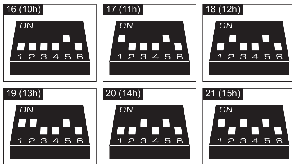
Рис. 21. Способ установки адресов в считывателях INT-IT.
