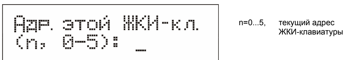
Рис. 8. Программирование адреса ЖКИ-клавиатуры с помощью сервисной функции.
