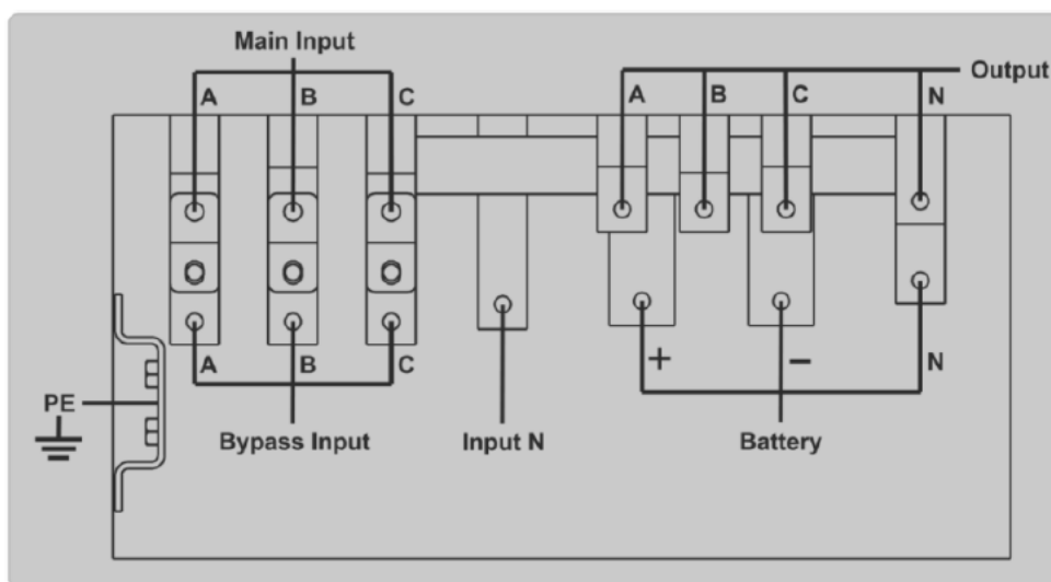
(б) Клеммы подключения ИБП 150/160 кВА и 200 кВА
