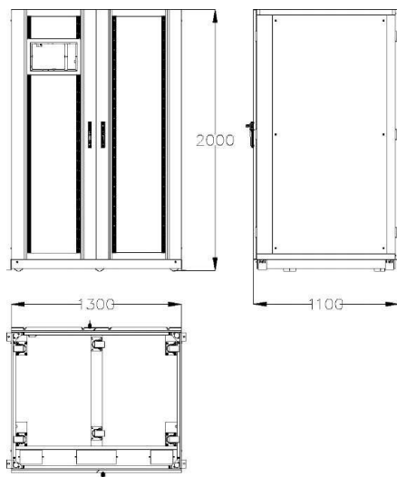
(е) Размеры ИБП 400 кВА и 500 кВА (размеры в миллиметрах) Рисунок 2-2. Размеры Рис. 3-2 Размеры ИБП
