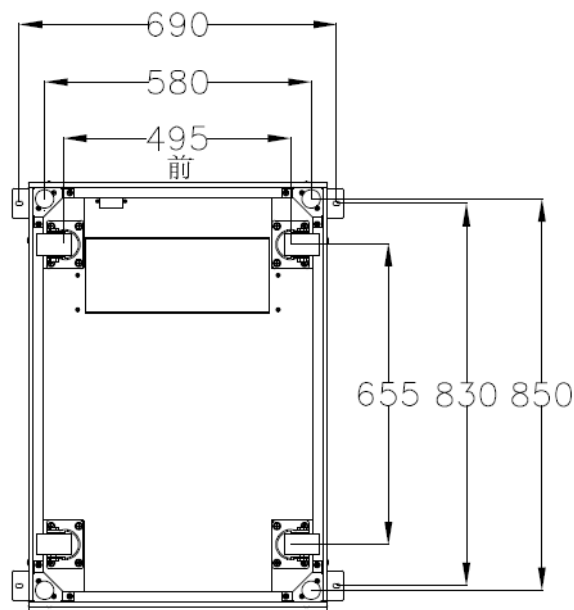
(е) Опорная конструкция ИБП 150/160 кВА и 200 кВА, 250 кВА и 300 кВА (вид снизу, размеры в миллиметрах)
