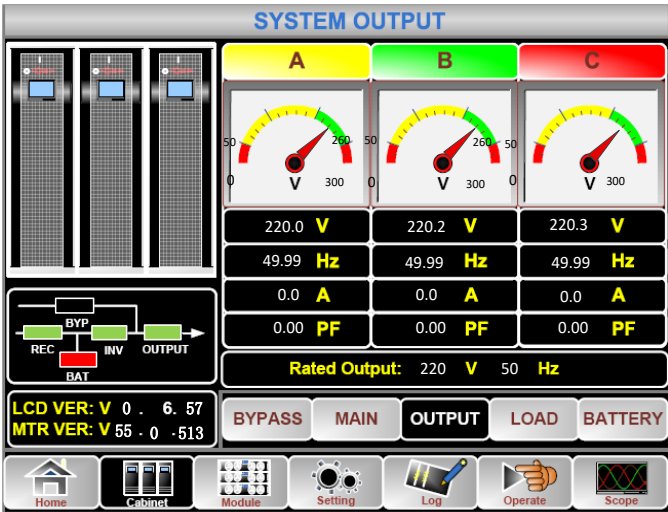
Рисунок 4-5(б) Интерфейс подменю «Выход»
