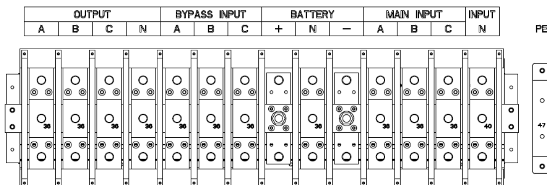
(г) Клеммы подключения ИБП 400 кВА и 500 кВА
