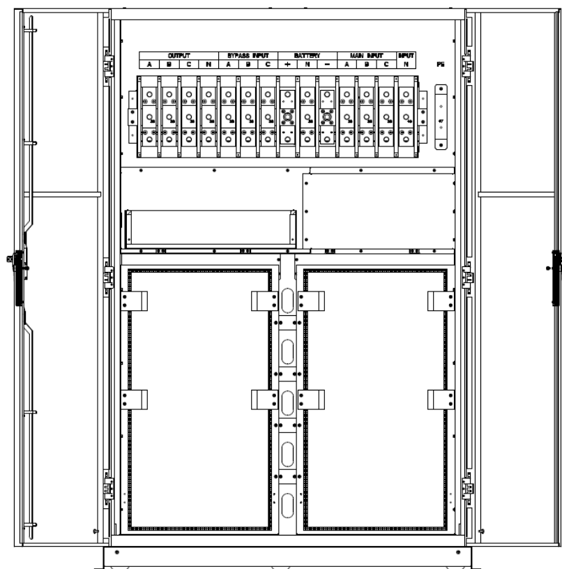
(е) Конструкция ИБП 400 кВА и 500 кВА Рис 2-7 Конструкция ИБП
