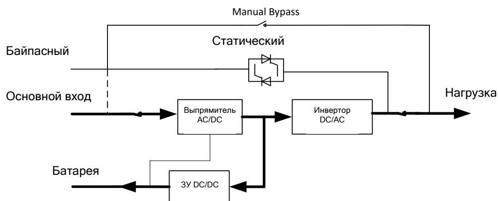
Рисунок 2-2 Структурная схема работы ИБП в нормальном режиме
