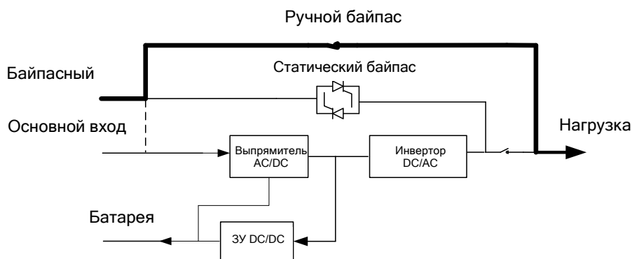
Рисунок 2-5 Структурная схема ИБП в режиме обслуживания
