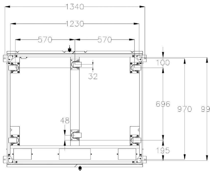
(е) Опорная конструкция ИБП 400 кВА и 500 кВА (вид снизу, размеры в миллиметрах) Рисунок 3-6 Опорная конструкция
