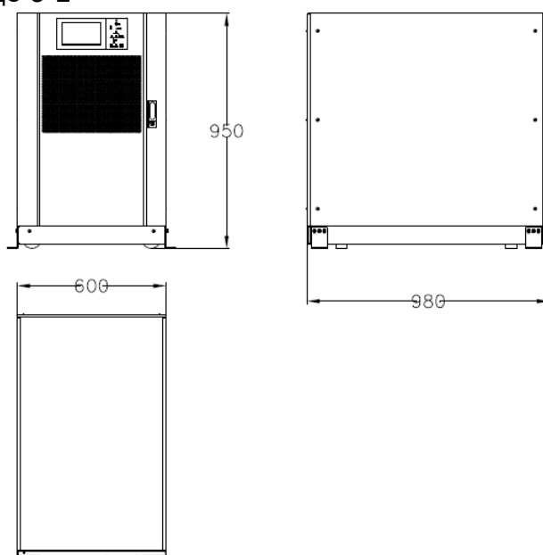
(а) Размеры ИБП 60 кВА (размеры в миллиметрах)
