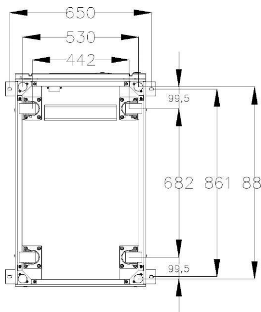
(б) Опорная конструкция ИБП 80 кВА и 100 кВА (вид снизу, размеры в миллиметрах)
