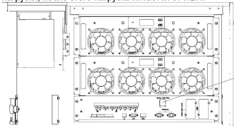
Рисунок 5-1. Расположение кнопки холодного пуска аккумулятора
