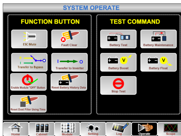
Рисунок 4-10 Меню «Управление»
