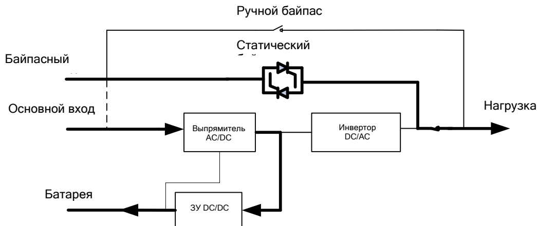
Рисунок 2-6 Структурная схема ИБП в ЭКО-режиме
