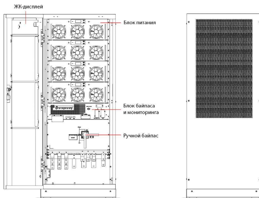
(г) Конструкция ИБП 150/160 кВА и 200 кВА
