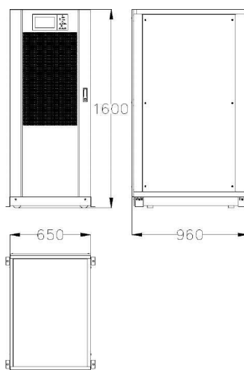
(г) Размеры ИБП 150/160 кВА и 200 кВА (размеры в миллиметрах)
