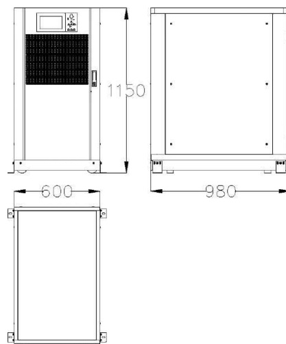
(в) Размеры ИБП 80 кВА и 100 кВА (размеры в миллиметрах)
