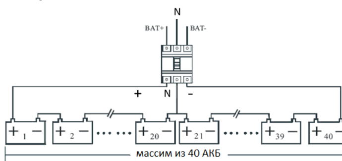
Рисунок 3-7 Схема подключения батарей
