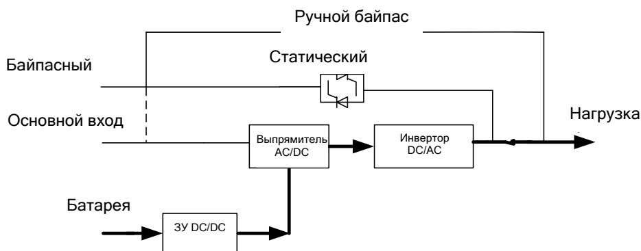
Рисунок 2-3 Структурная схема работы ИБП в режиме от АКБ
