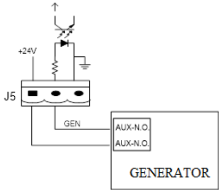
Рисунок 3-19 Порт подключения генератора
