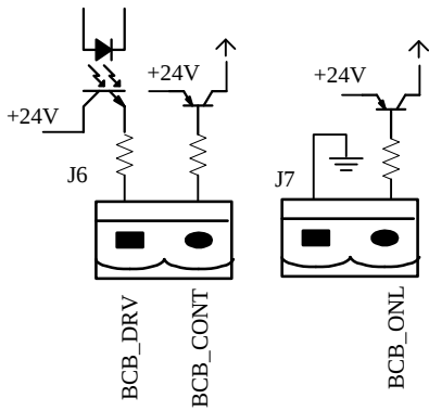
Рисунок 3-20 BCB порт
