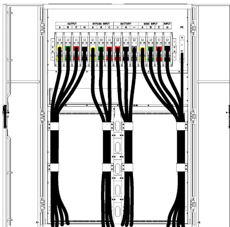
(г) Ввод кабелей снизу для ИБП 400 кВА и 500 кВА Рисунок 3-8. Ввод кабелей
