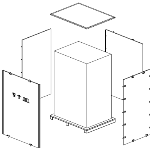
Рис 3-4 Снятие упаковки
