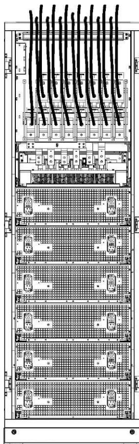
(б) Ввод кабелей для ИБП 250 кВА-300 кВА
