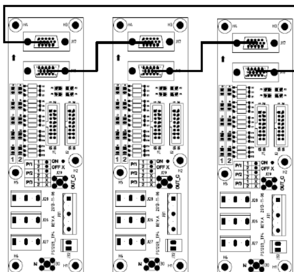
Рисунок 5-8 Схема подключения кабелей параллельной работы
