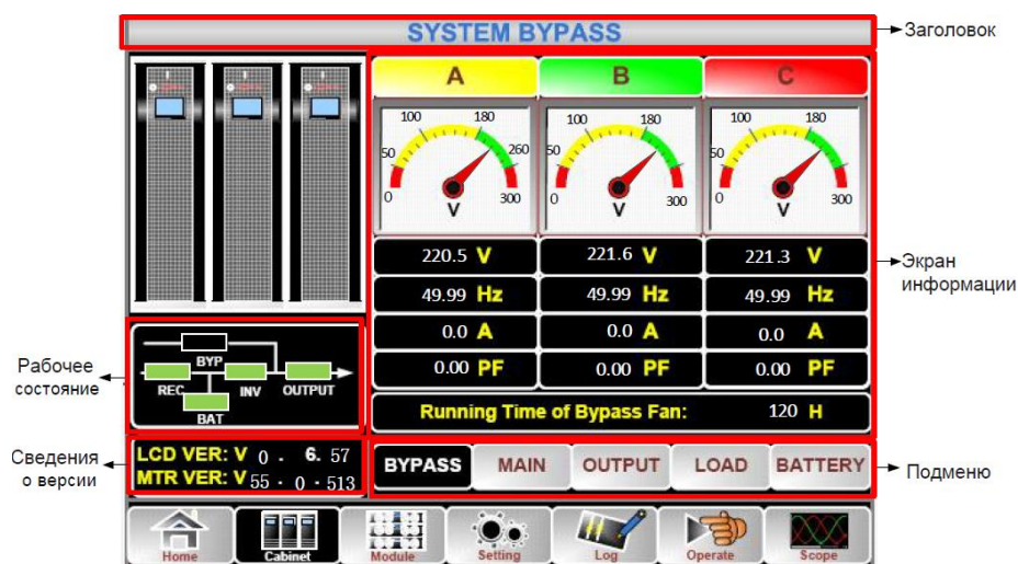
Рисунок 4-4. Меню «Кабинет»
