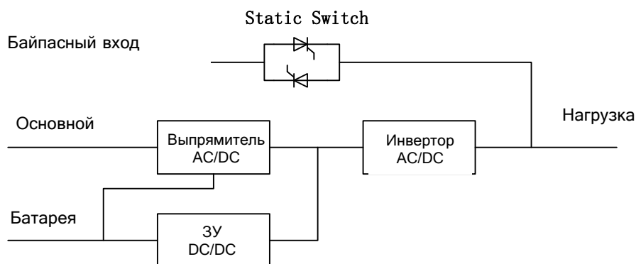
Рис. 2-1 Структурная схема ИБП
