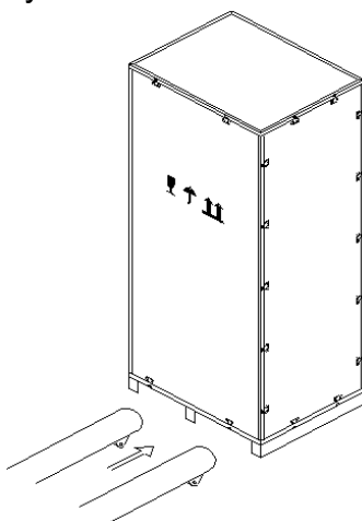
Рис 3-3 Способ перемещения шкафа ИБП
