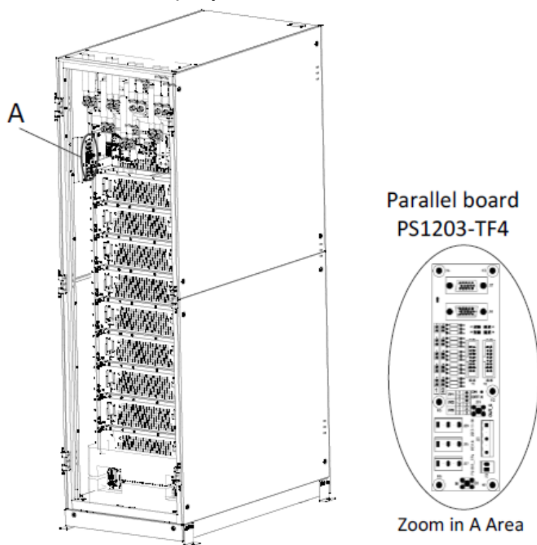
Рисунок 5-7 (а) Терминал параллельной работы
