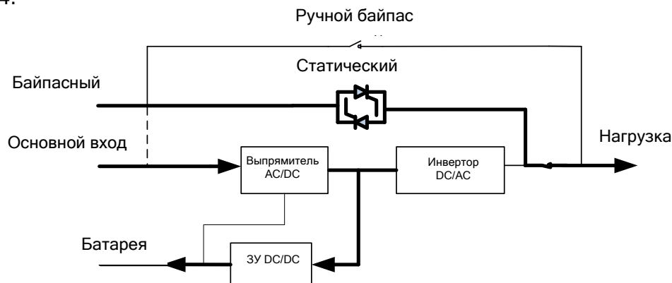
Рисунок 2-4 Структурная схема ИБП в режиме байпаса
