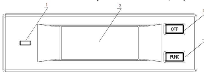
1-Индикатор статуса; 2-LCD-экран; 3-Кнопка выключения силового модуля; 4-Функциональная кнопка Рисунок 4-1 Схема пользовательской панели
