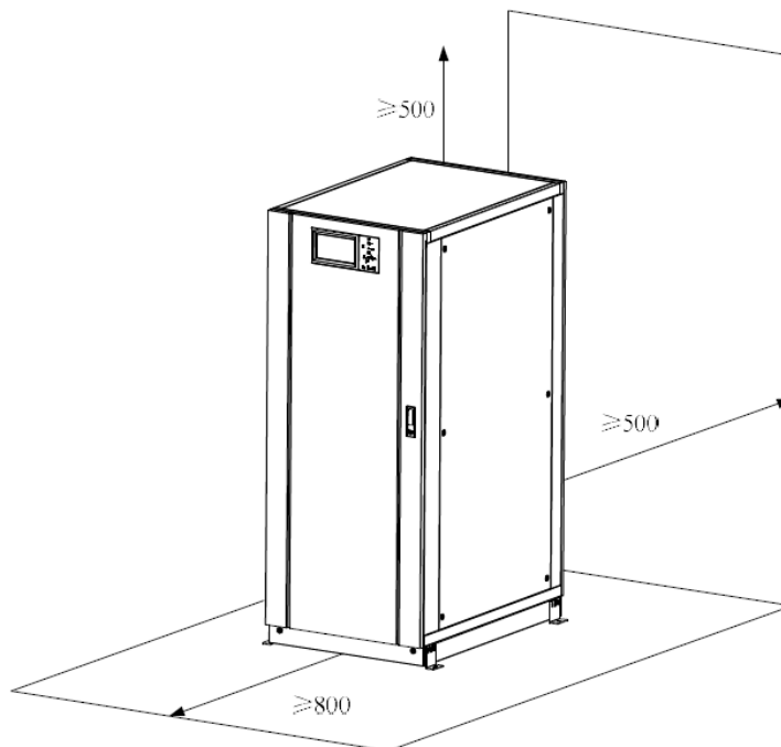
Рис 3-1 Размеры помещения для ИБП
