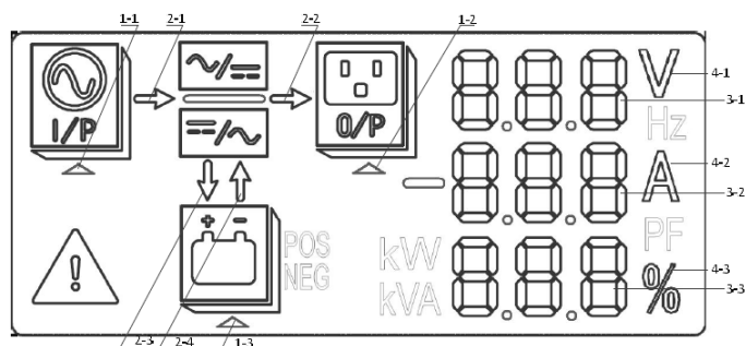
1: Треугольник выбора параметра, 2: Направление энергии 3: область отображения цифр 4: Параметр
