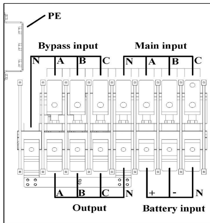
(в) Клеммы подключения ИБП 250 кВА и 300 кВА
