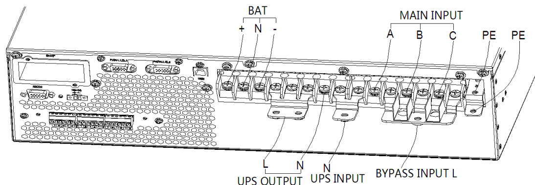
Рис. 3-18 3 фазы в 1 фазу, двойной вход
