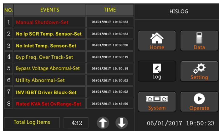
Рис. 4-5 Страница «Журнал событий»
