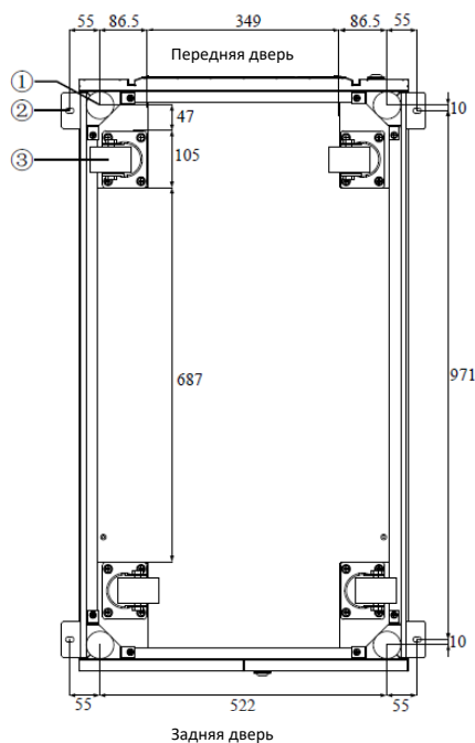
Рисунок 3-8 (а) Несущая конструкция ИБП для 6-10 силовых модулей
