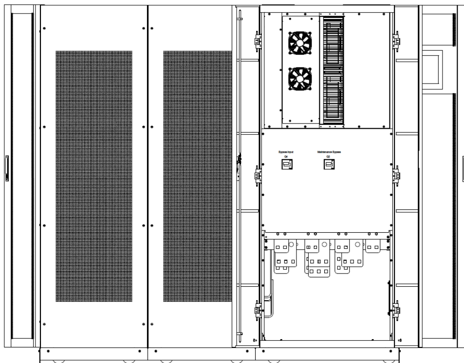
Рисунок 2-10(в) Задняя сторона ИБП для 20 силовых модулей
