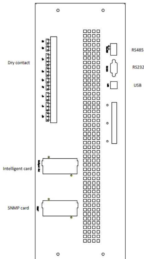
Рисунок 3-16 (б) Расположение интерфейсов для 20-ти модульного ИБП
