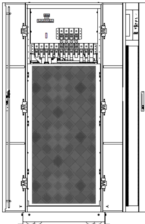
Рисунок 2-10(а) Задняя сторона ИБП для 6 силовых модулей
