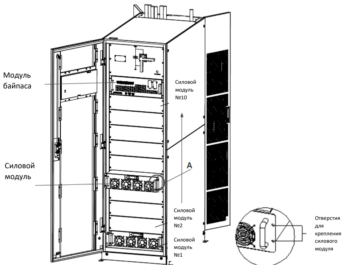
Рисунок 3-9 Установка силовых модулей
