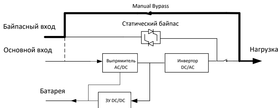
Рисунок 2-6 Структурная схема ИБП в режиме обслуживания
