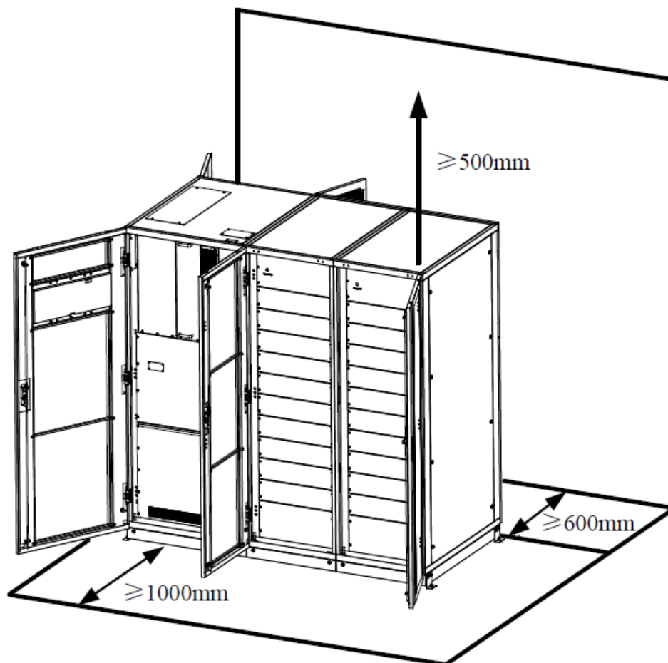
Рисунок 3-1(в) Размеры помещения для ИБП из 20 силовых модулей (мм)
