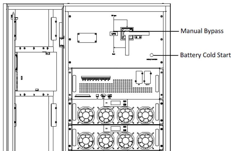
Рисунок 5-1(а) Кнопка холодного запуска для 10-ти модульного ИБП
