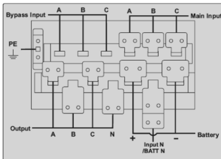
Рисунок 3-12 (б) Клемма 10-ти модульного ИБП
