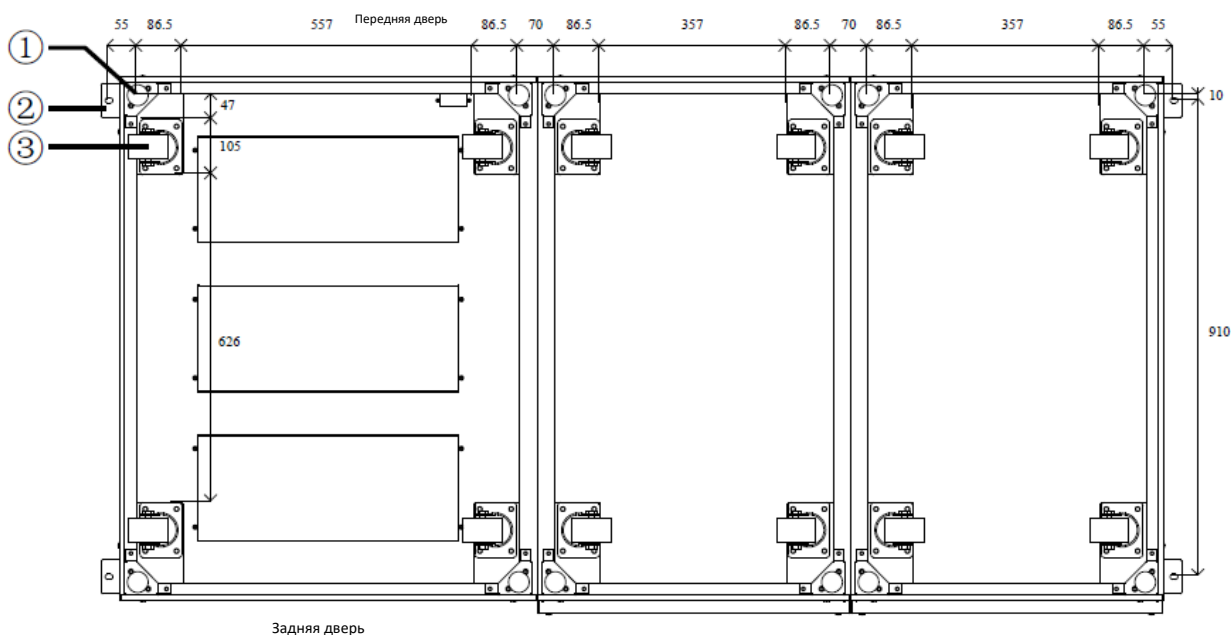
Рисунок 3-8 (а) Несущая конструкция ИБП для 6-10 силовых модулей
