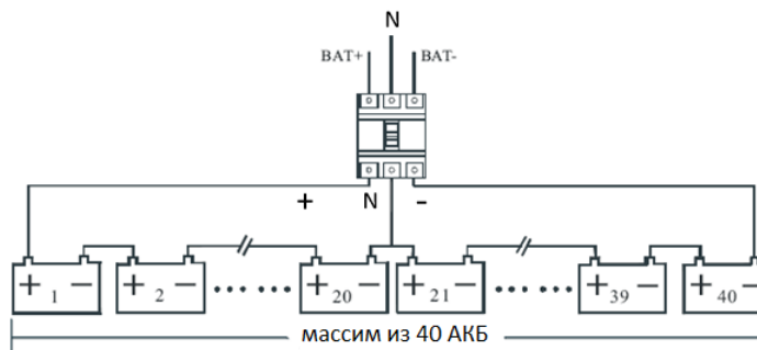
Рисунок 3-10 Схема подключения батарей
