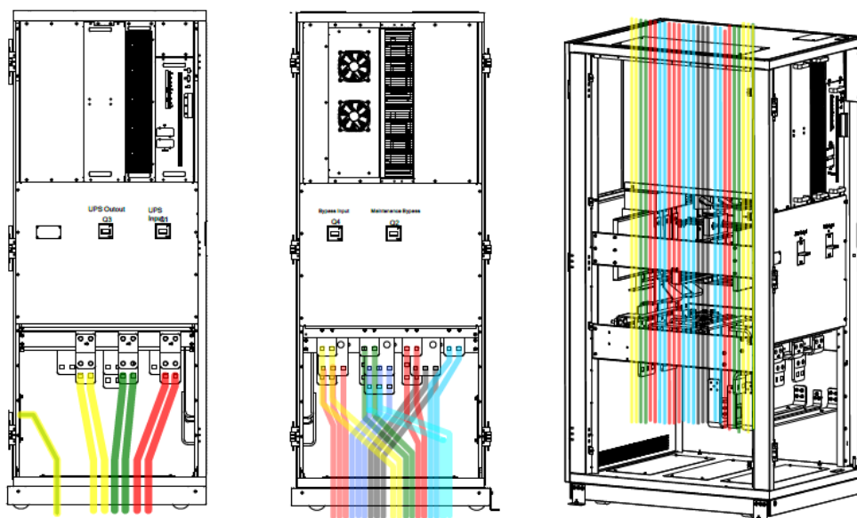
Рисунок 3-11 (в) Подвод кабелей для 10-ти модульного ИБП
