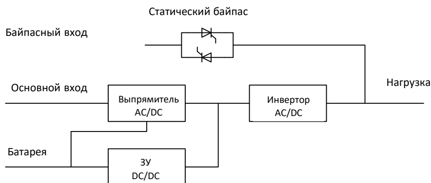
Рисунок Ошибка! Текст указанного стиля в документе отсутствует. -1(а) Структурная схема 6-ти и 10-ти модульного ИБП
