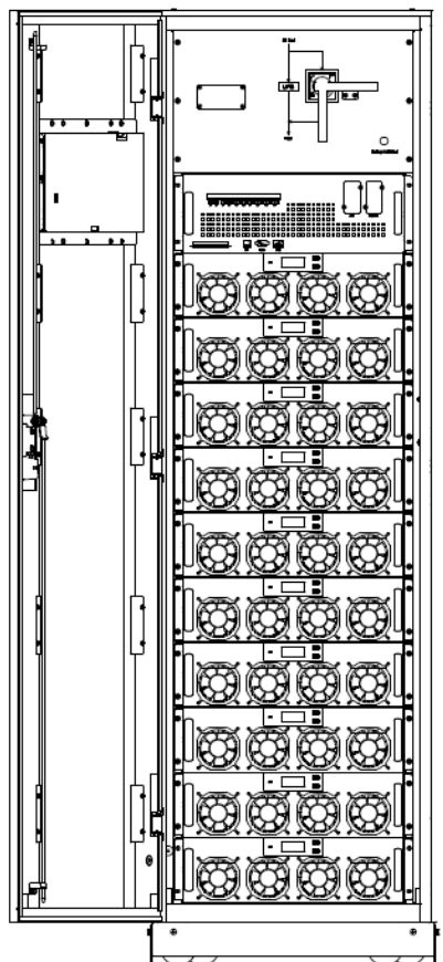
Рисунок 2-9(б) Вид спереди ИБП для 10 силовых модулей
