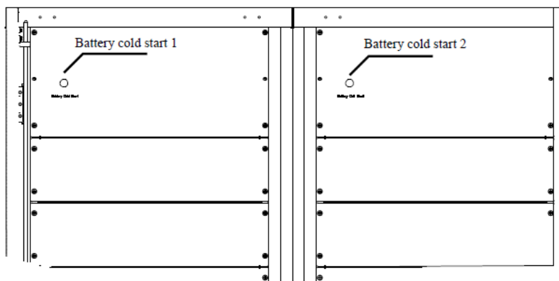
Рисунок 5-2(б) Кнопка холодного запуска для 20-ти модульного ИБП
