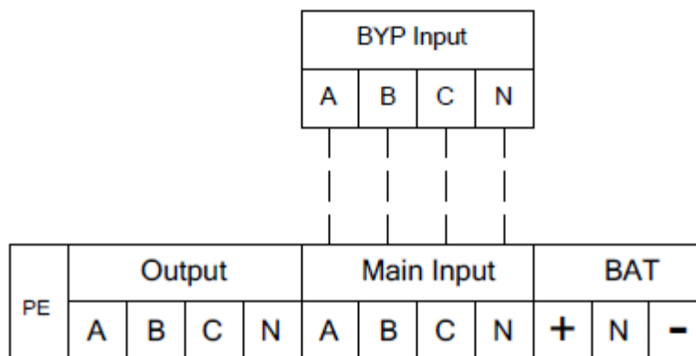
Рисунок 3-12 (а) Клемма 6-ти модульного ИБП
