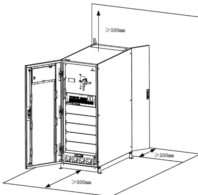
Рисунок 3-1(а) Размеры помещения для ИБП из 6 силовых модулей (мм)
