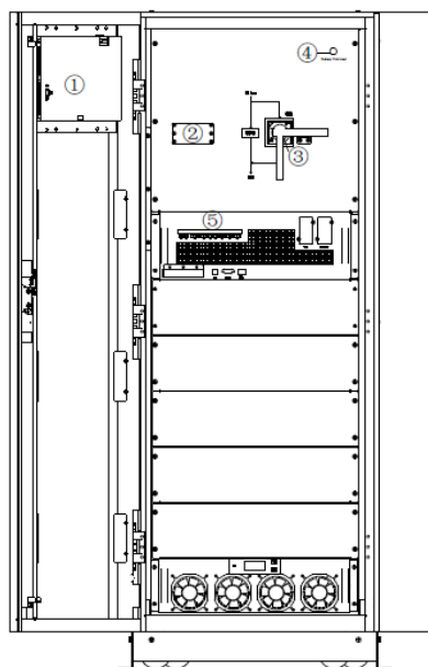
Рисунок 2-9(а) Вид спереди ИБП для 6 силовых модулей
