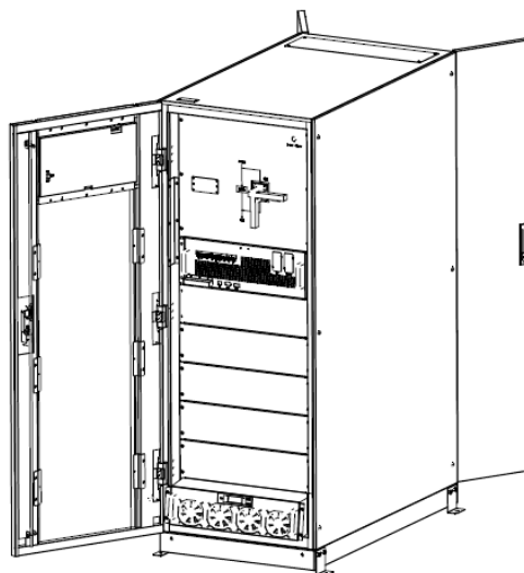
Рисунок 2-8(а) Структура ИБП для 6 силовых модулей
