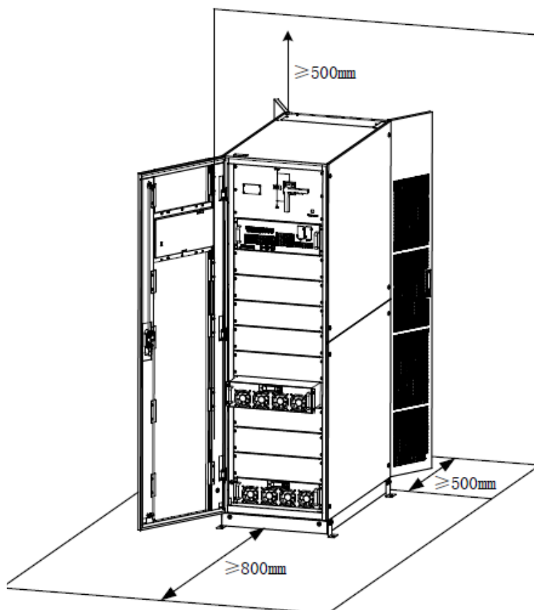
Рисунок 3-1(б) Размеры помещения для ИБП из 10 силовых модулей (мм)
