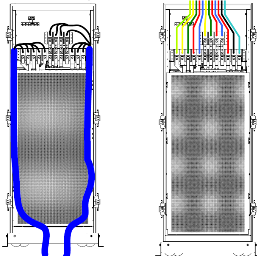
Рисунок 3-11 (а) Подвод кабелей для 6-ти модульного ИБП
