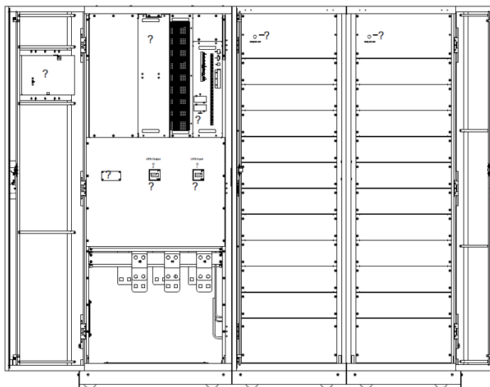
Рисунок 2-9(в) Вид спереди ИБП для 20 силовых модулей
