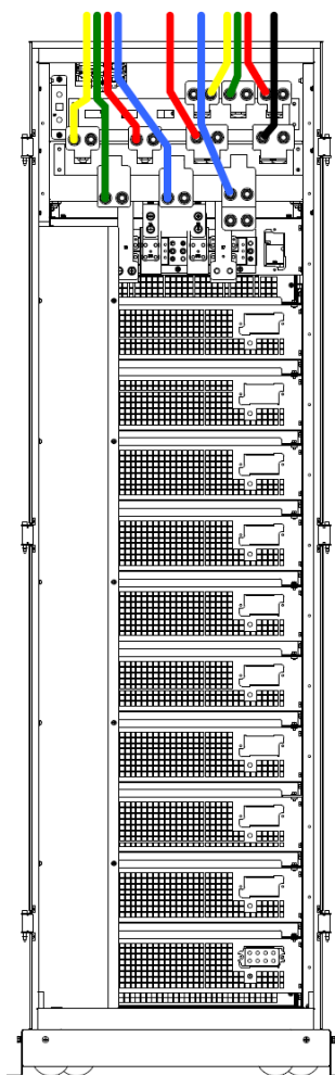
Рисунок 3-11 (б) Подвод кабелей для 10-ти модульного ИБП
