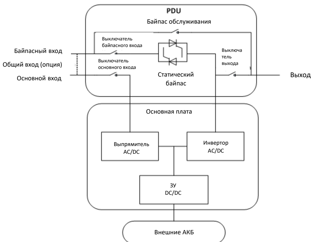
Рисунок Ошибка! Текст указанного стиля в документе отсутствует. -1(а) Структурная схема 6-ти и 10-ти модульного ИБП
