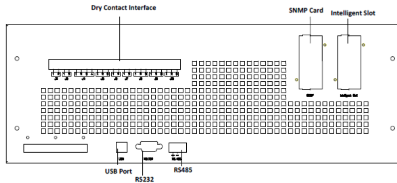
Рисунок 3-13 (а) Расположение интерфейсов 6-ти и 10-ти модульного ИБП
