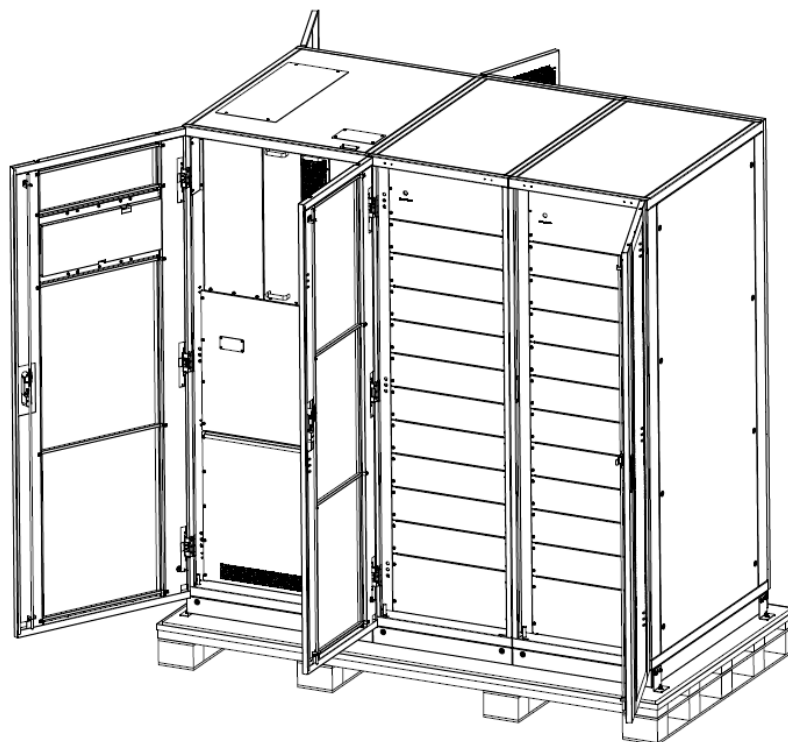
Рисунок 2-8(в) Структура ИБП для 20 силовых модулей
