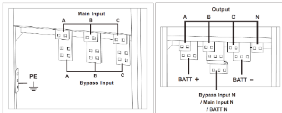
Рисунок 3-12 (в) Клемма 20-ти модульного ИБП
