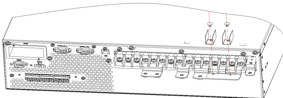
Рисунок 21. Установка изоляционной планки
