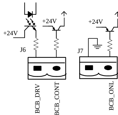
Рисунок 16. Контроль ВСВ (управление автоматическим выключателем АКБ)
