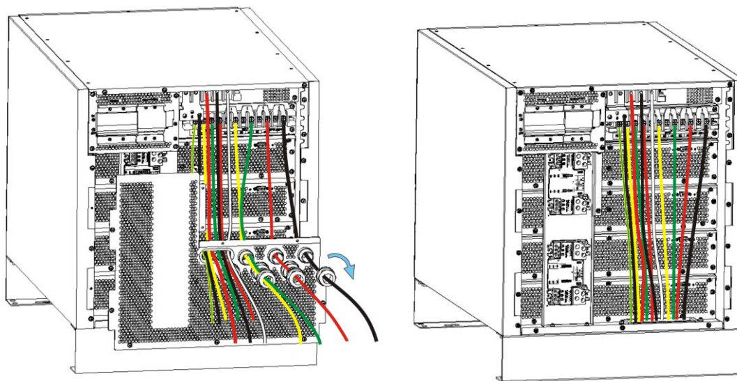
Рисунок 3-9 (а) Подвод кабелей к 2-4 х модульному ИБП
