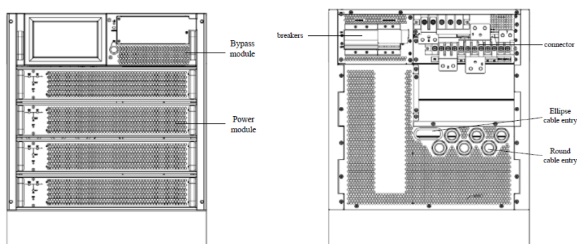
Рисунок 2-8(б) Структура ИБП для 4 силовых модулей
