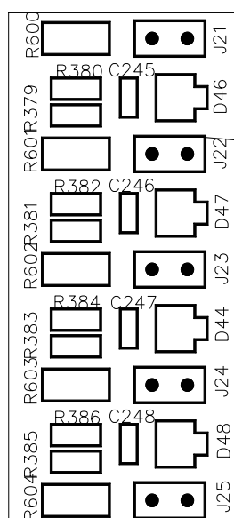
Рисунок 5-12 Плата контроля (PS1203_СТ1)
