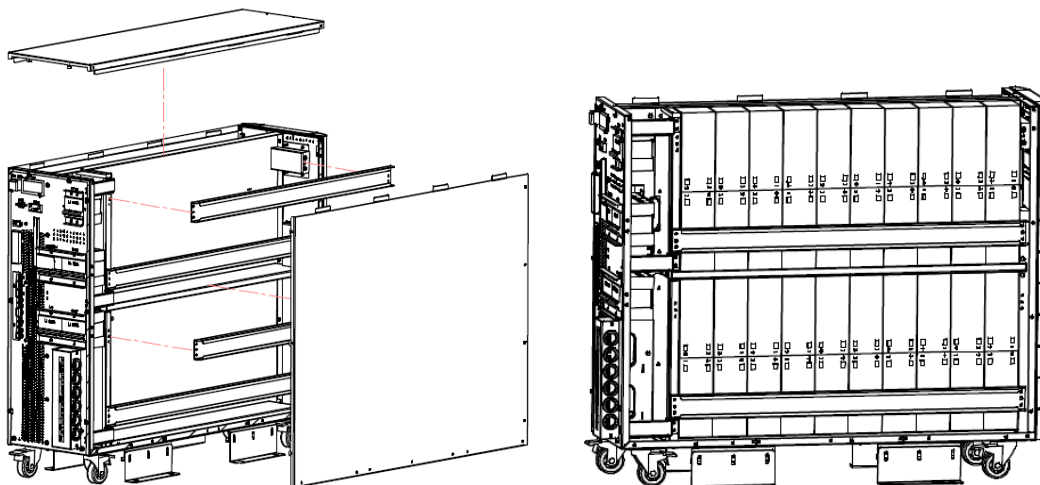
1. Снятие крышек и фиксирующих планок
