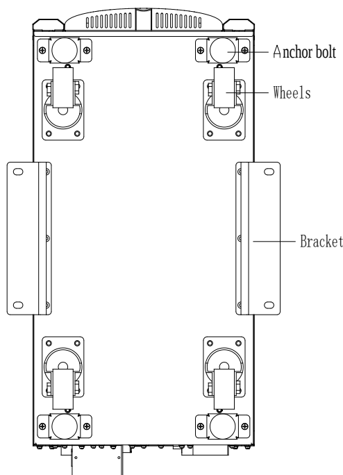
Рисунок.3-8 Вид снизу на транспортные ролики и фиксирующие ИБП ножки
