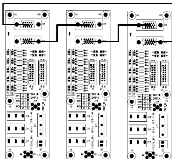
Рисунок 5-8 Схема подключения кабелей параллельной работы
