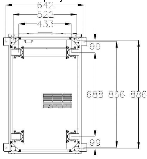
(а) Опорная конструкция ИБП 60 кВА, 90 кВА и 120 кВА (вид снизу, размеры в миллиметрах)
