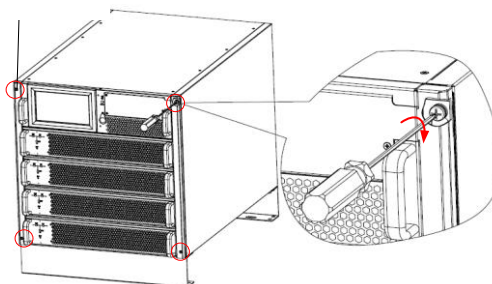
Рисунок 3-6 (б) Установка декоративной планки
