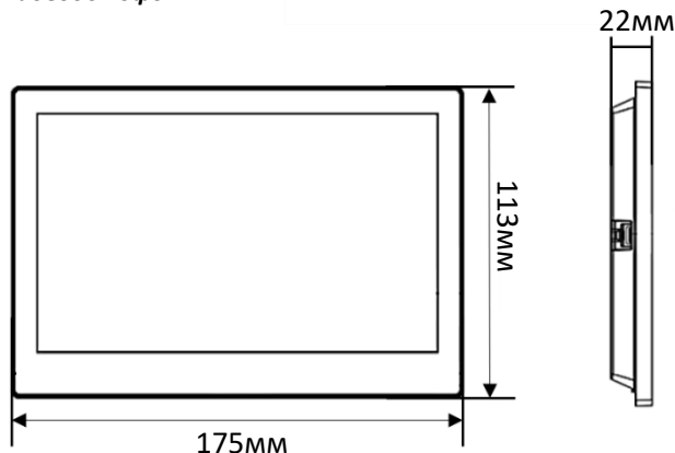
Видеодомофон
