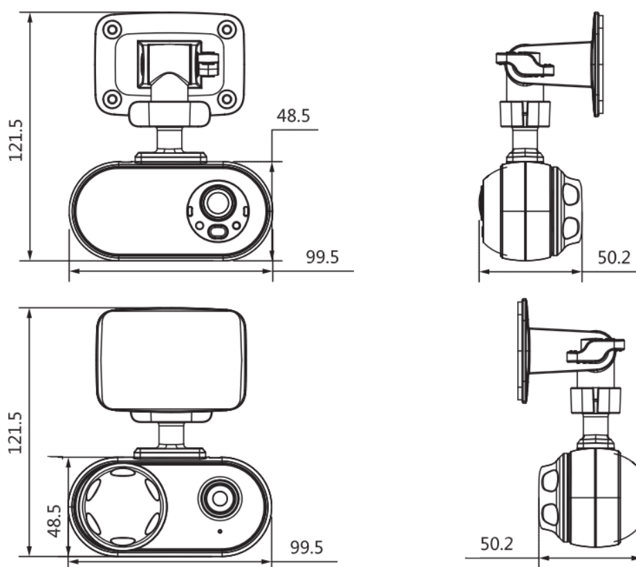
Рисунок 5.1 – Габаритные размеры видеокамеры
