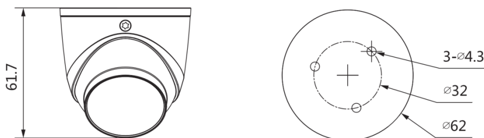
Рисунок 5.1 – Габаритные размеры видеокамеры
