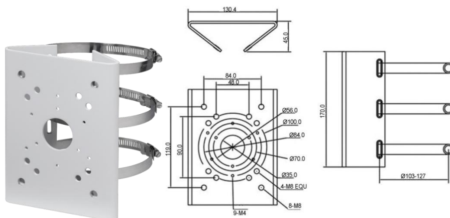
Рисунок 5.10 – Столбовой кронштейн BR-103
