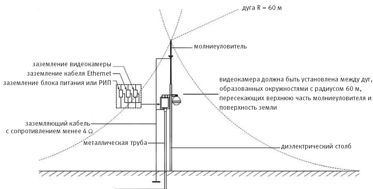
Рисунок 6.6 – Установка молниеотвода
