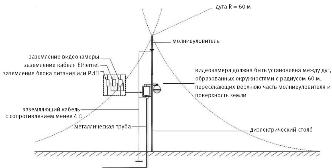
Рисунок 8.4 – Установка молниеотвода
