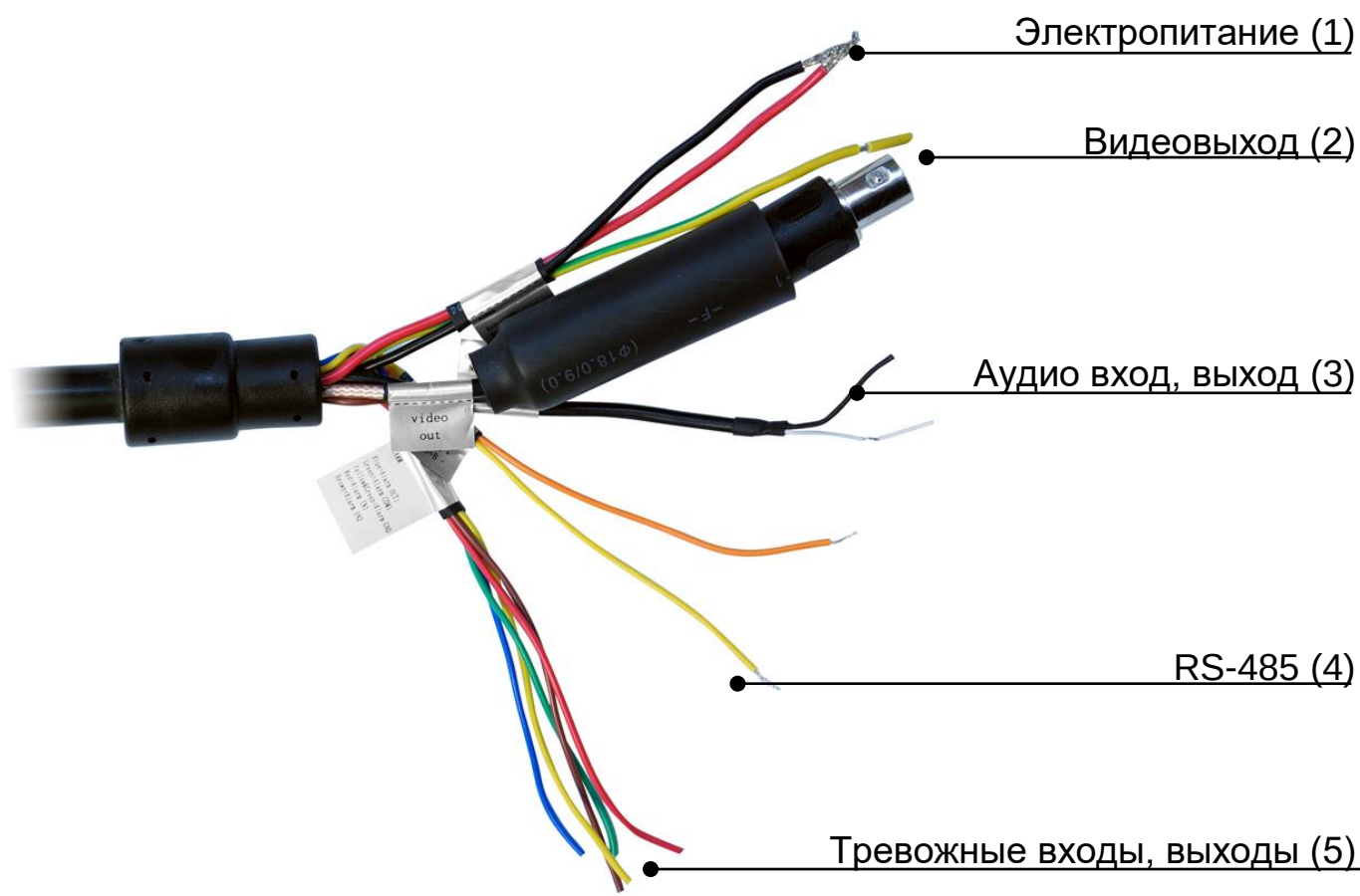
Рисунок 6.1 – Группы концевой раскладки кабеля видеокamеры
