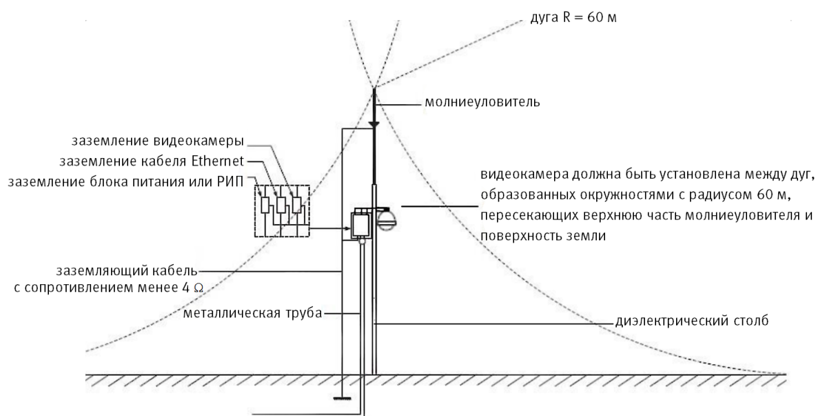
Рисунок 6.6 – Установка молниеотвода
