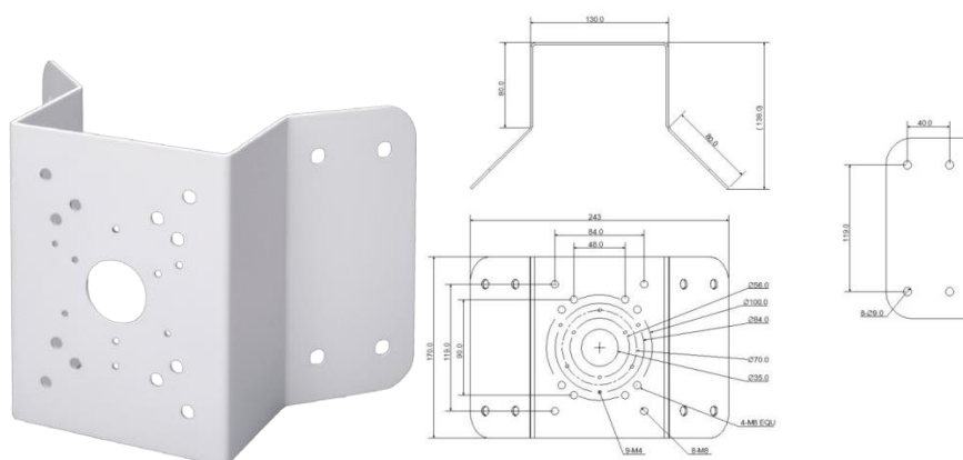
Рисунок 5.7 – Угловой кронштейн BR-102
