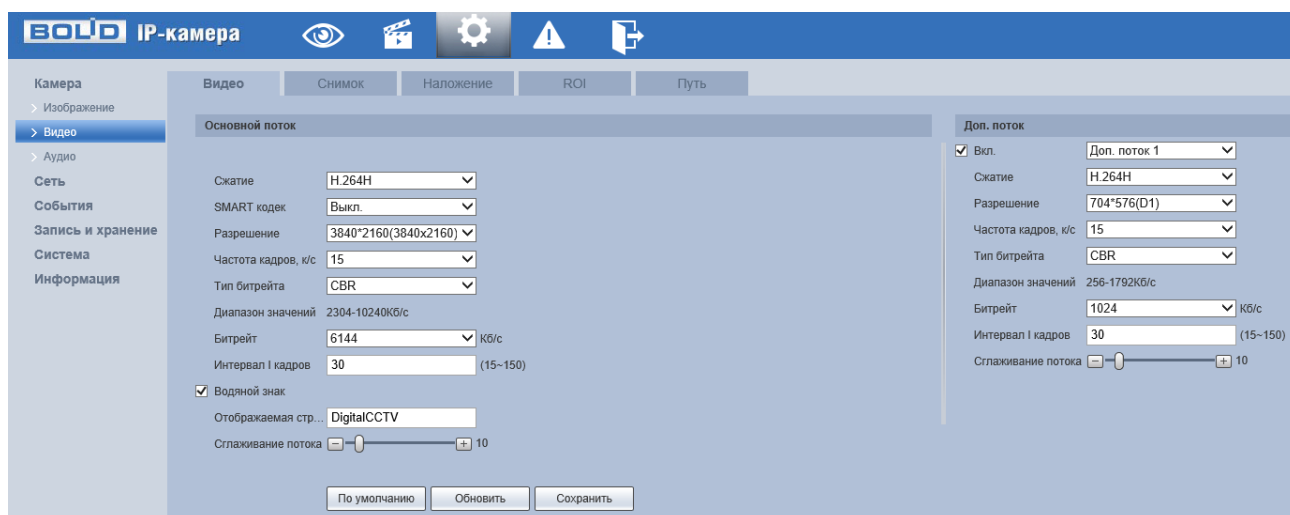
Рисунок 7.38 – Вкладка «Видео»
