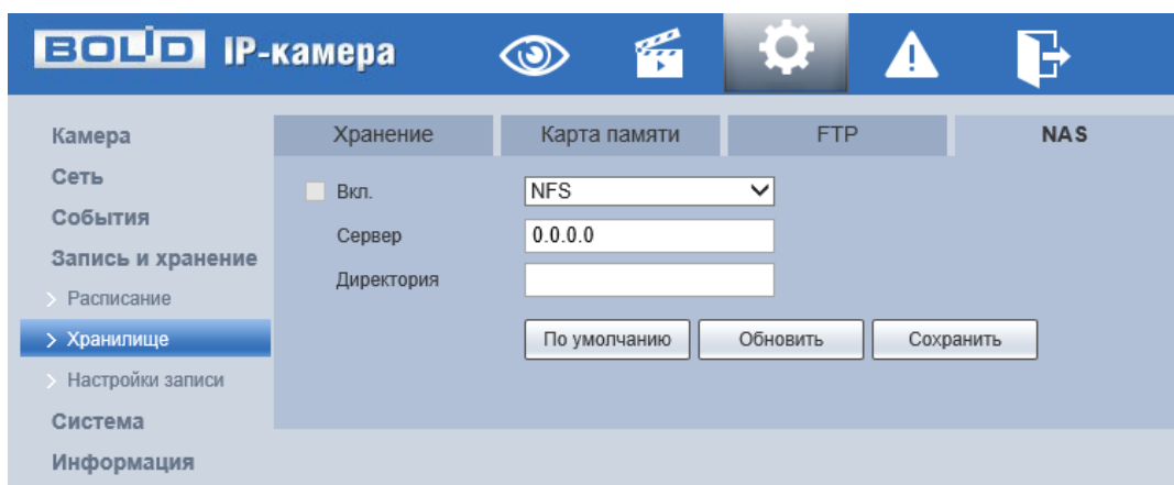
Рисунок 7.108 – Вкладка «NAS»
