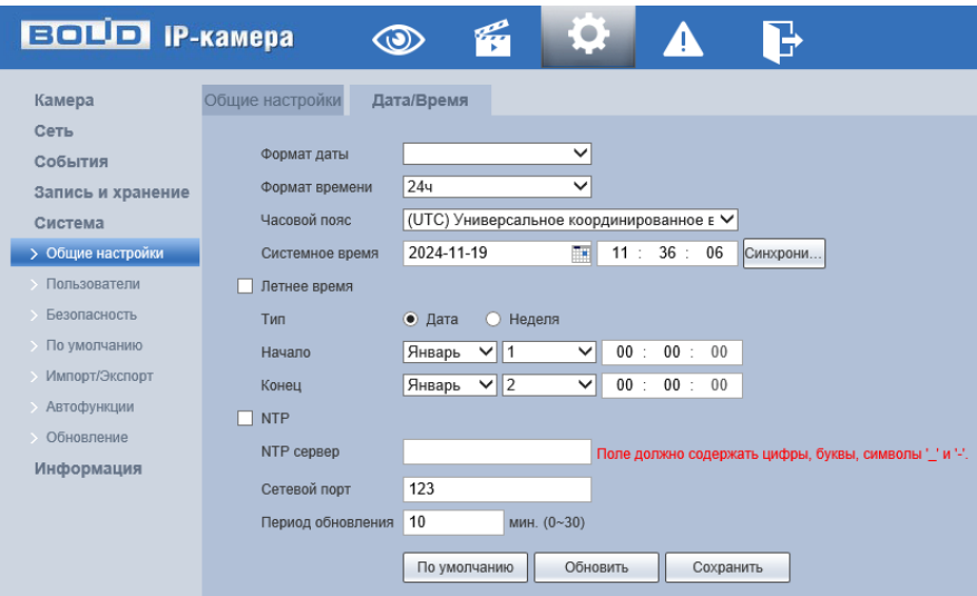
Рисунок 7.114 – Вкладка «Дата/Время»
