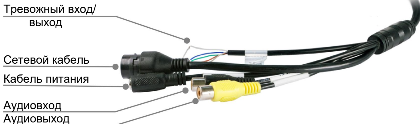
Рисунок 6.1 – Кабель видеокamеры
