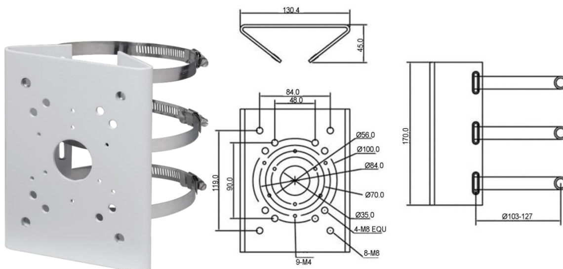
Рисунок 5.11 – Столбовой кронштейн BR-103
