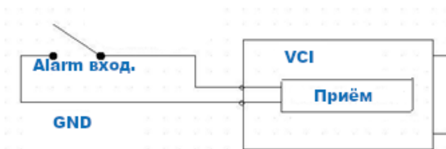
Рисунок 6.13 – Схема подключения тревожного входа
