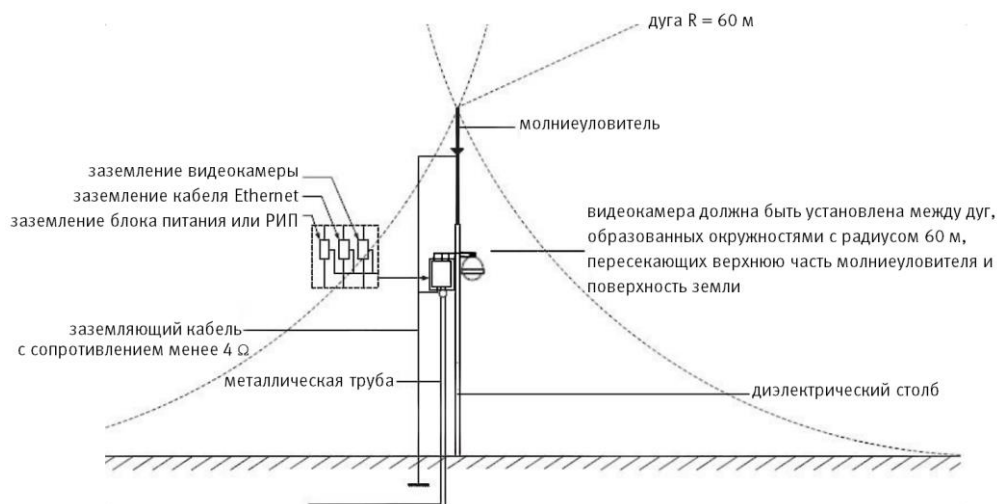
Рисунок 6.14 – Установка молниеотвода
