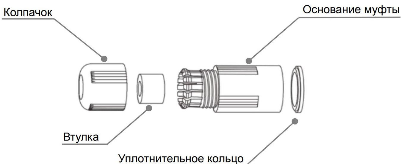
Рисунок 6.6 – Элементы герметичной кабельной муфты
