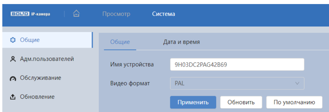
Рисунок 7.104 – Вкладка «Общие»
