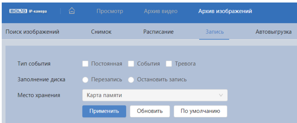
Рисунок 7.136 – Вкладка «Запись»
