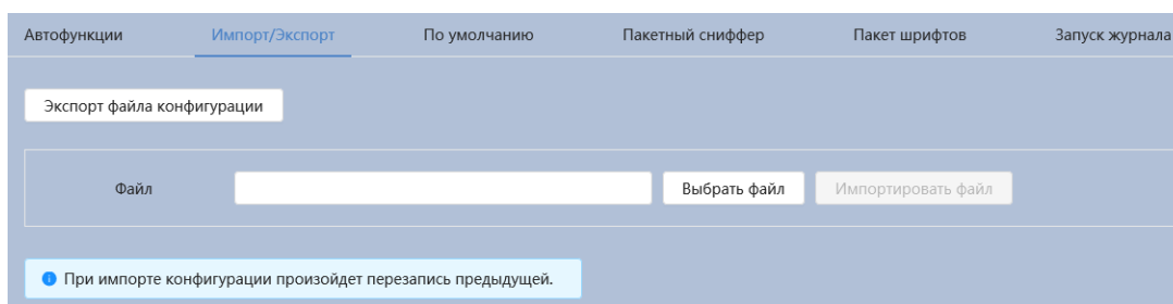
Рисунок 7.117 – Вкладка «Импорт/Экспорт»
