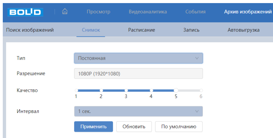
Рисунок 7.133 – Вкладка «Снимок»
