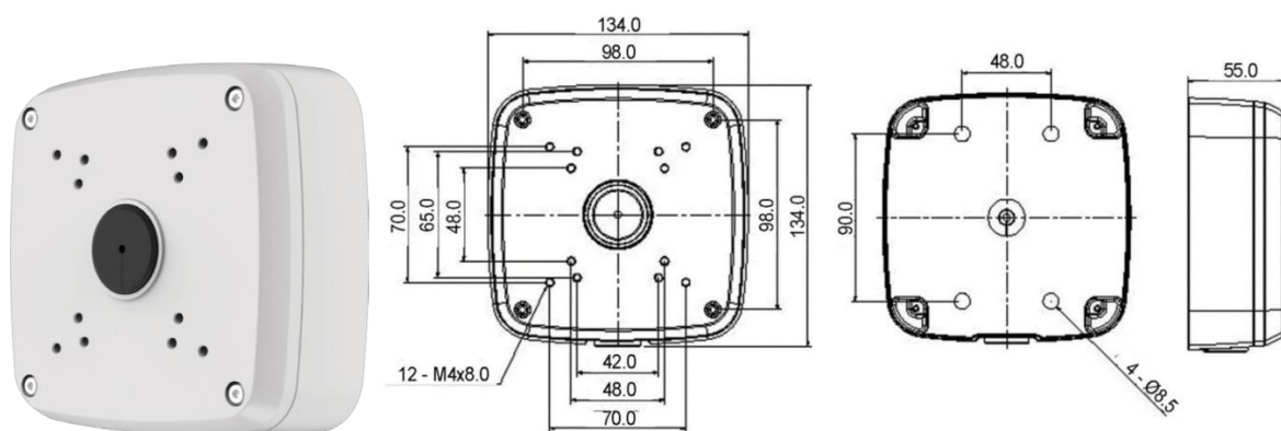
Рисунок 5.3 – Монтажная коробка BR-201
