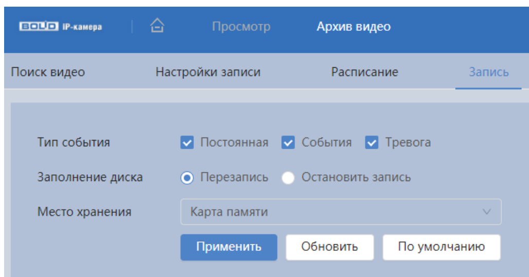
Рисунок 7.130 – Вкладка «Запись»
