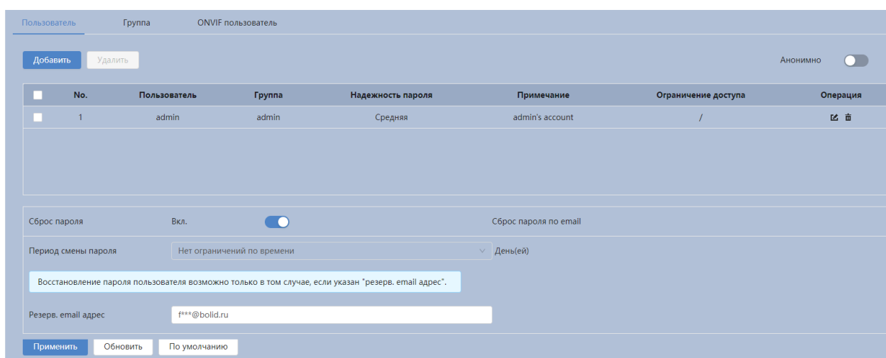
Рисунок 7.107 – Вкладка «Пользователь»
