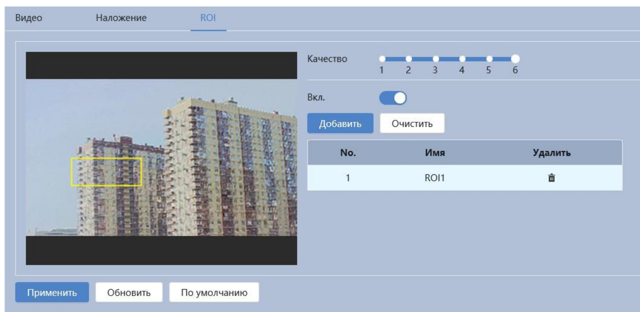
Рисунок 7.80 – Вкладка «ROI»
