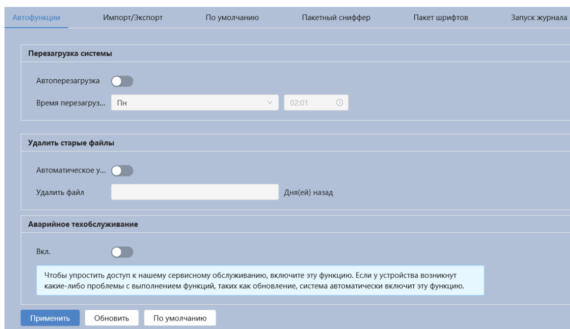
Рисунок 7.116 – Вкладка «Автофункции»
