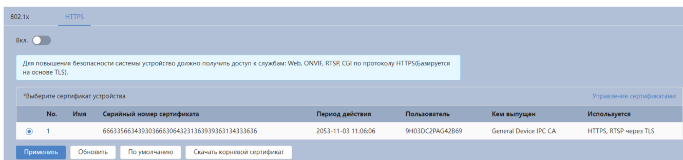
Рисунок 7.149 – Вкладка «HTTPS»
