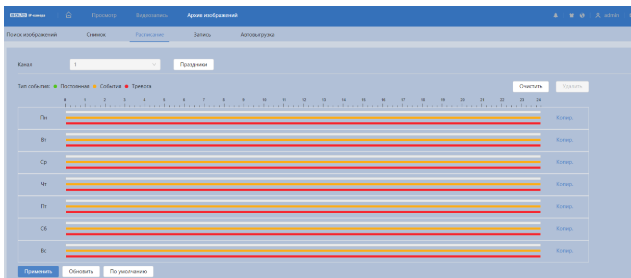
Рисунок 7.134 – Вкладка «Расписание»
