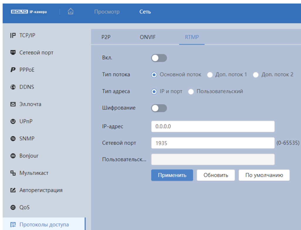
Рисунок 8.21 – Вкладка «RTMP»
