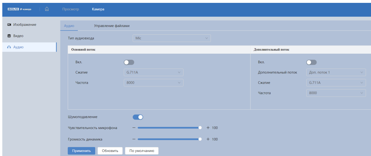
Рисунок 7.82 – Вкладка «Аудио»
