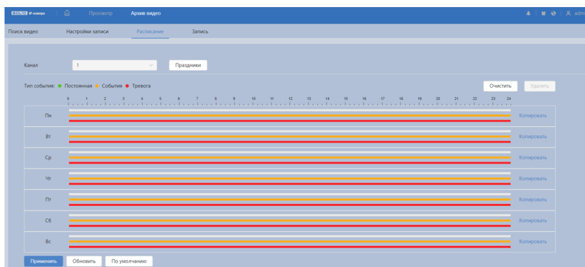
Рисунок 7.128 – Вкладка «Расписание»
