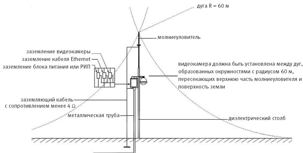
Рисунок 6.13 – Установка молниеотвода
