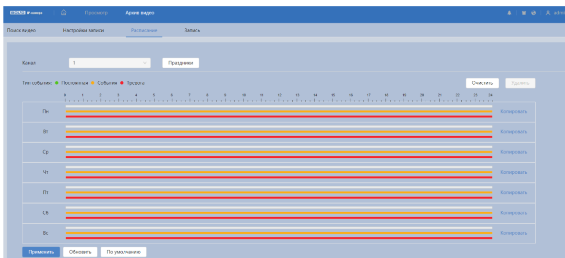
Рисунок 7.131 – Вкладка «Расписание»
