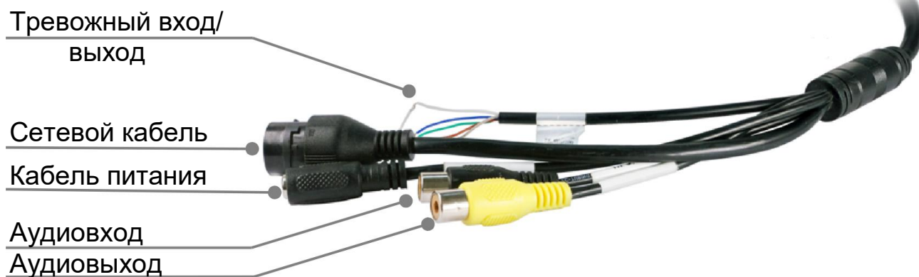
Рисунок 6.1 – Кабель видеокмеры
