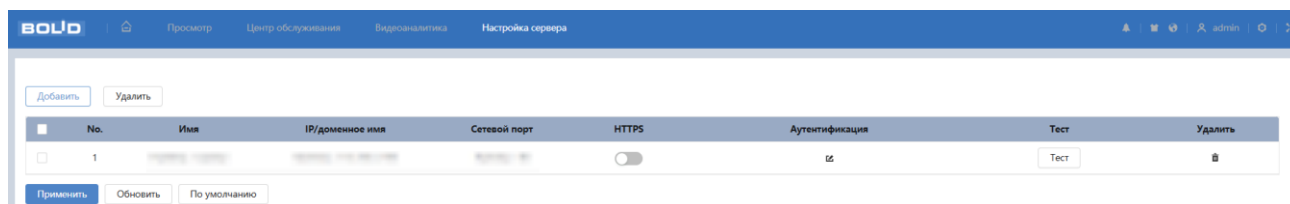
Рисунок 7.26 – Настройка сервера
