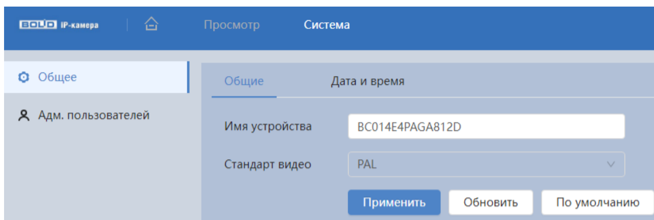
Рисунок 7.115 – Вкладка «Общие»
