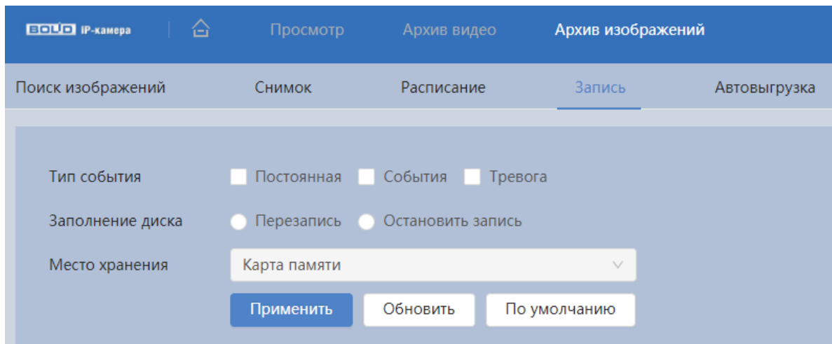
Рисунок 7.139 – Вкладка «Запись»
