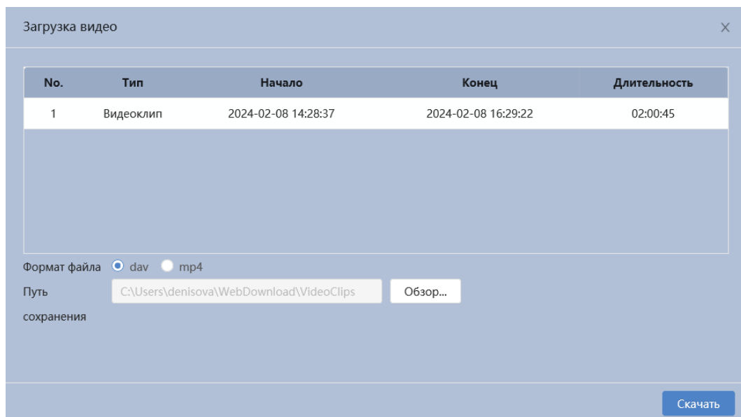
Рисунок 7.129 – Загрузка видео
