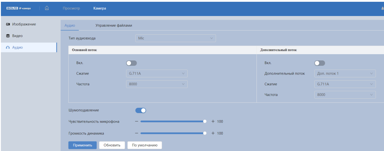
Рисунок 7.90 – Вкладка «Аудио»
