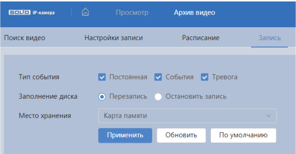
Рисунок 7.133 – Вкладка «Запись»
