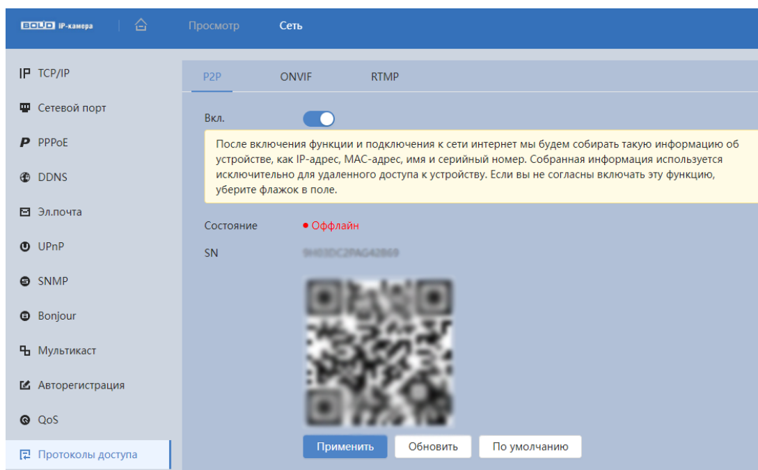
Рисунок 8.19 – Вкладка «P2P»
