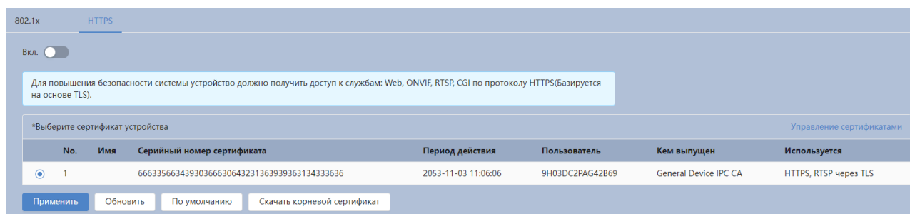
Рисунок 7.144 – Вкладка «HTTPS»
