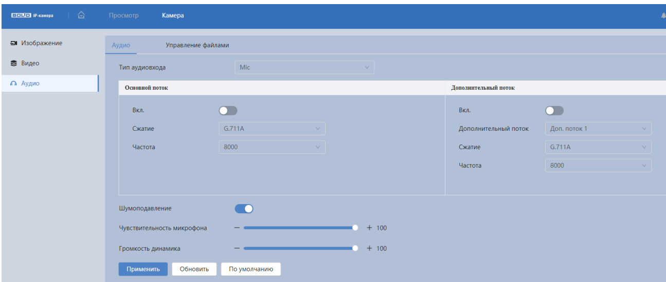
Рисунок 7.82 – Вкладка «Аудио»
