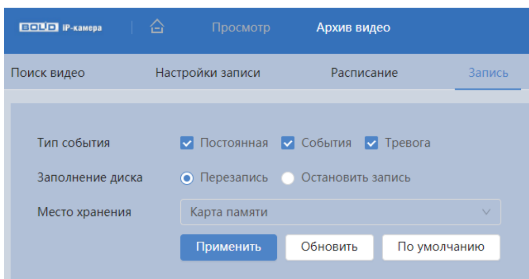
Рисунок 7.125 – Вкладка «Запись»
