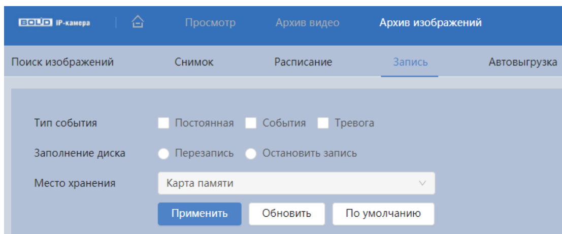
Рисунок 7.131 – Вкладка «Запись»
