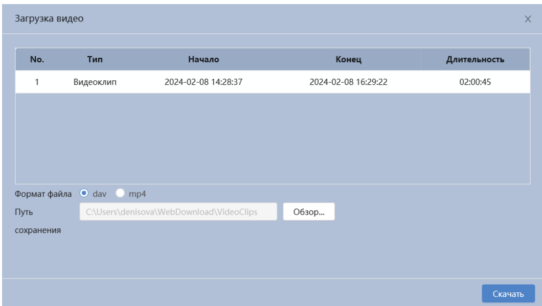
Рисунок 7.121 – Загрузка видео
