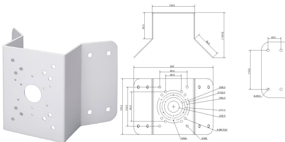
Рисунок 5.7 – Угловой кронштейн BR-102
