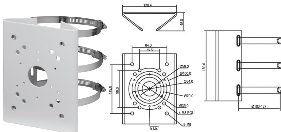
Рисунок 5.11 – Столбовой кронштейн BR-103
