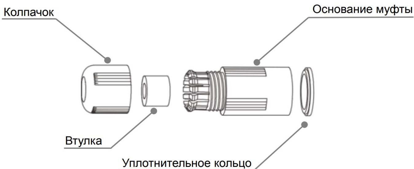
Рисунок 6.5 – Элементы герметичной кабельной муфты
