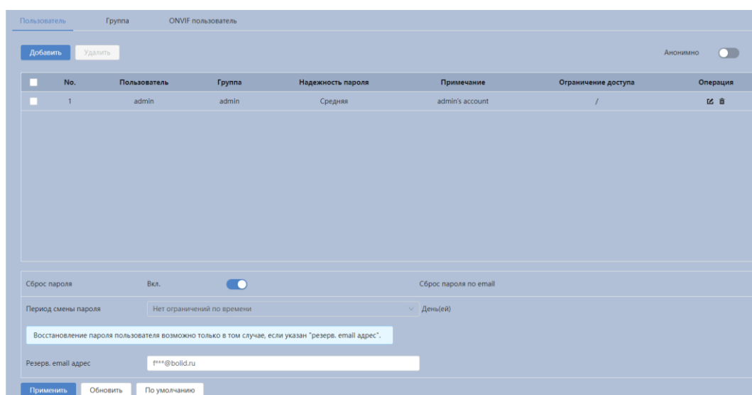
Рисунок 7.105 – Вкладка «Пользователь»
