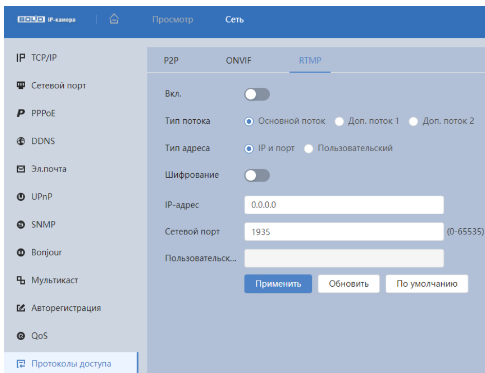
Рисунок 8.21 – Вкладка «RTMP»
