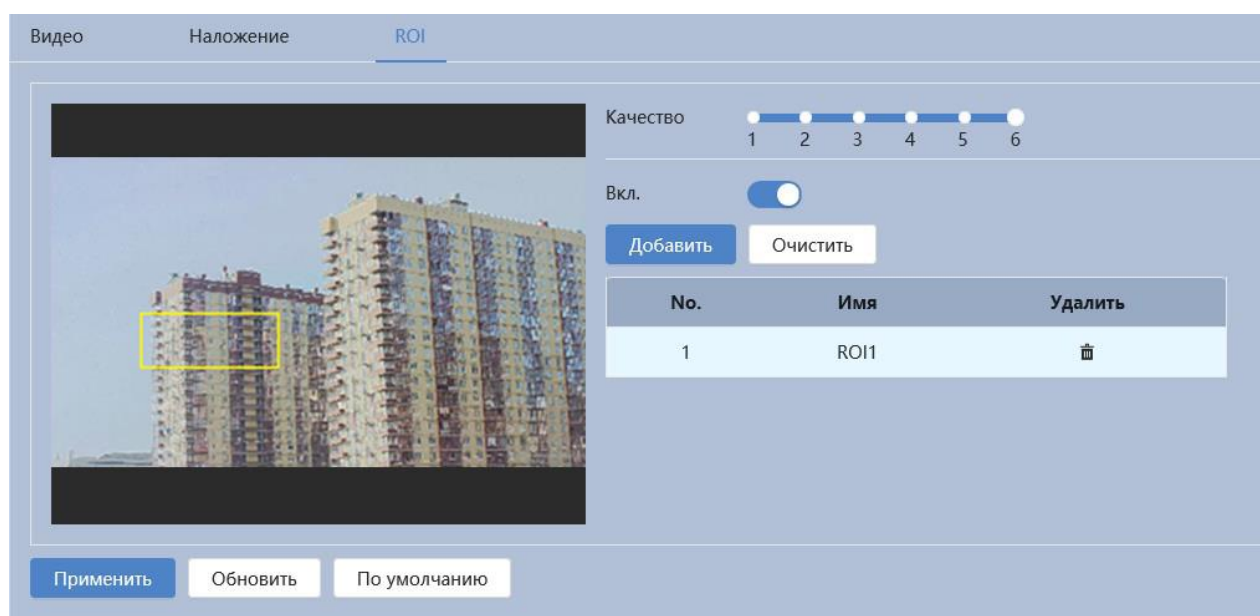
Рисунок 7.80 – Вкладка «ROI»
