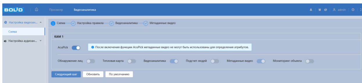
Рисунок 7.23 – Функция «АсиPick»
