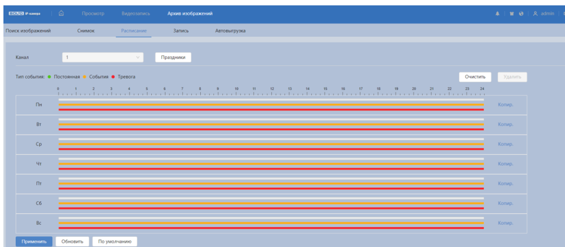
Рисунок 7.129 – Вкладка «Расписание»
