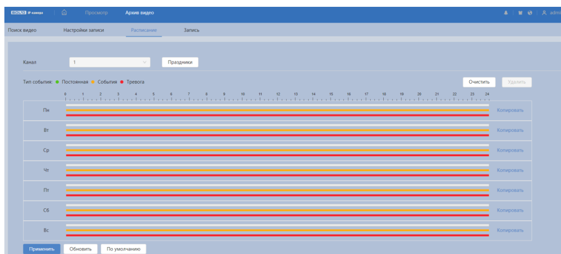
Рисунок 7.123 – Вкладка «Расписание»
