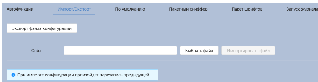
Рисунок 7.112 – Вкладка «Импорт/Экспорт»
