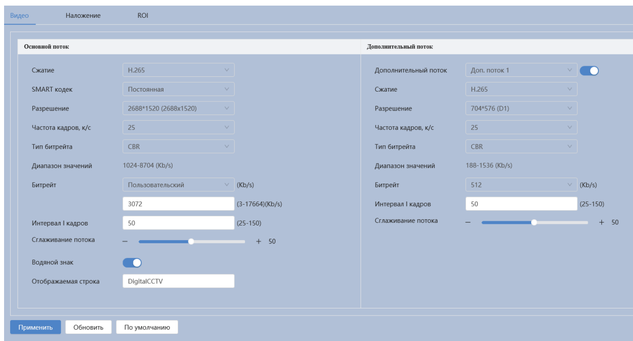
Рисунок 7.70 – Вкладка «Видео»
