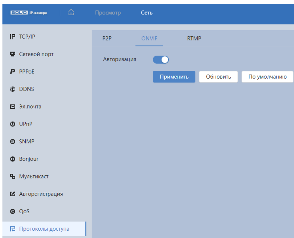
Рисунок 8.20 – Вкладка «ONVIF»
