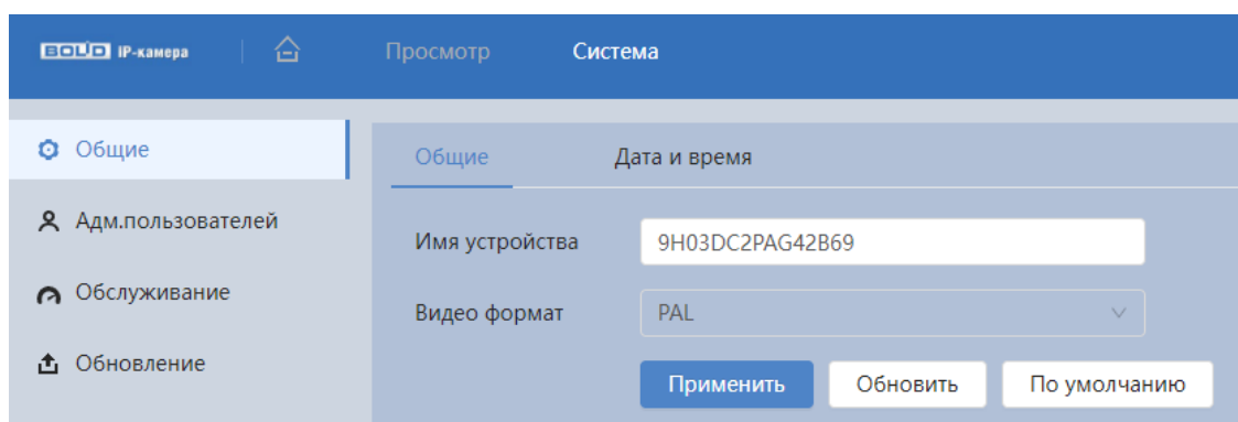
Рисунок 7.102 – Вкладка «Общие»
