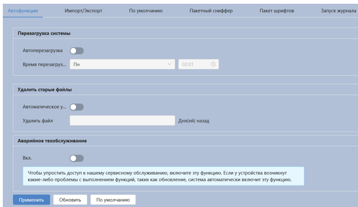
Рисунок 7.111 – Вкладка «Автофункции»
