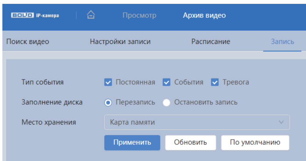
Рисунок 7.126 – Вкладка «Запись»
