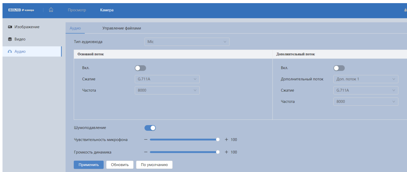
Рисунок 7.82 – Вкладка «Аудио»
