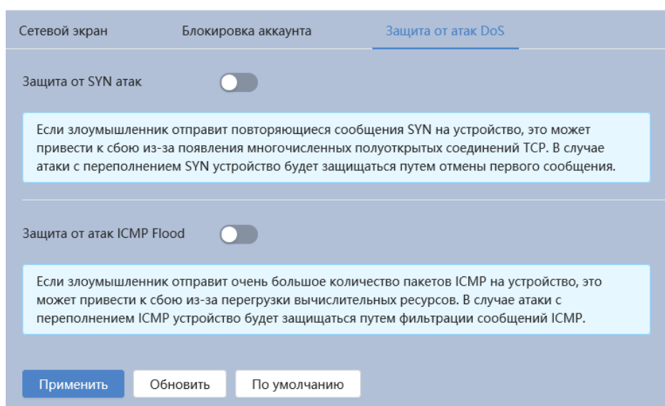
Рисунок 7.149 – Вкладка «Защита от атак DoS»
