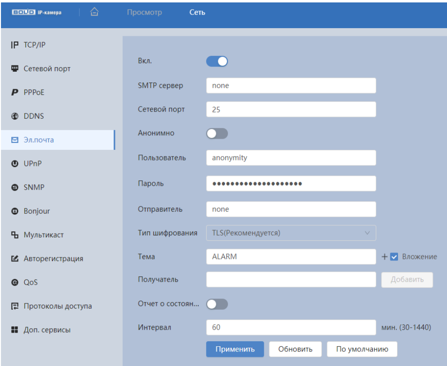
Рисунок 8.10 – Подпункт меню «Эл. почта»
