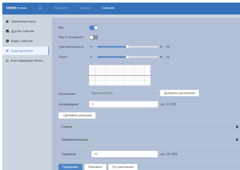
Рисунок 7.97 – Подраздел меню «Аудиодетекция»
