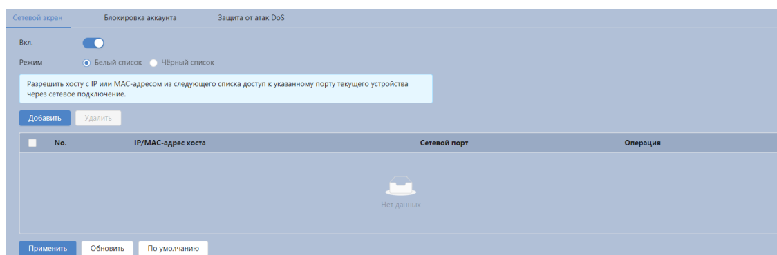
Рисунок 7.147 – Вкладка «Сетевой экран»
