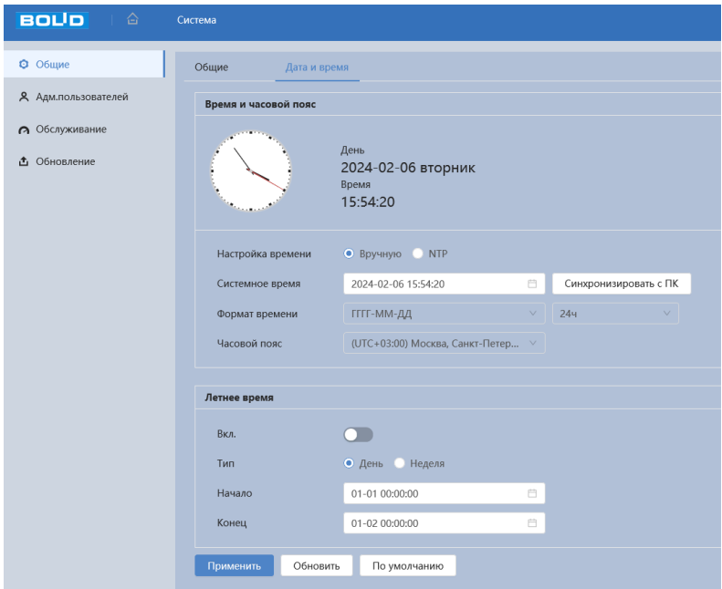
Рисунок 7.103 – Вкладка «Дата и время»
