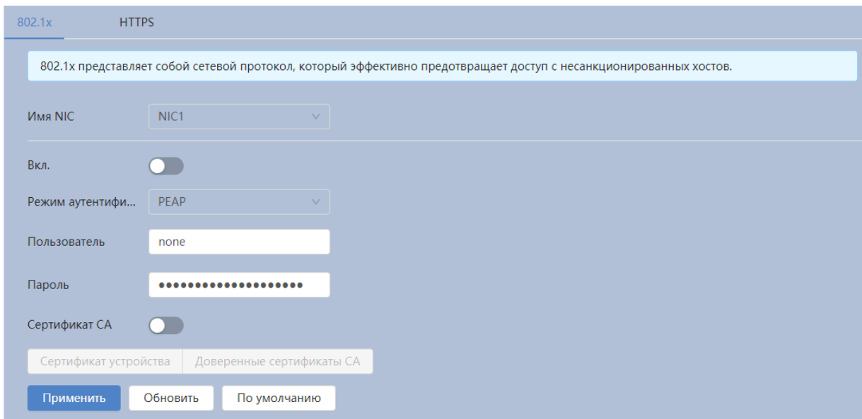
Рисунок 7.144 – Вкладка «Службы: 802.1x»
