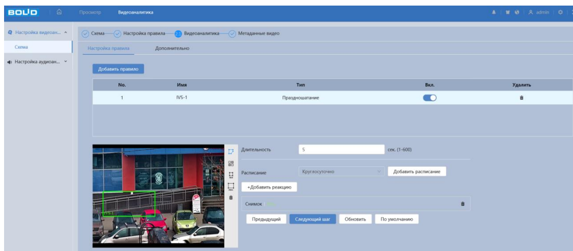
Рисунок 7.33 – Создание правила видеоаналитики «Праздношатание»
