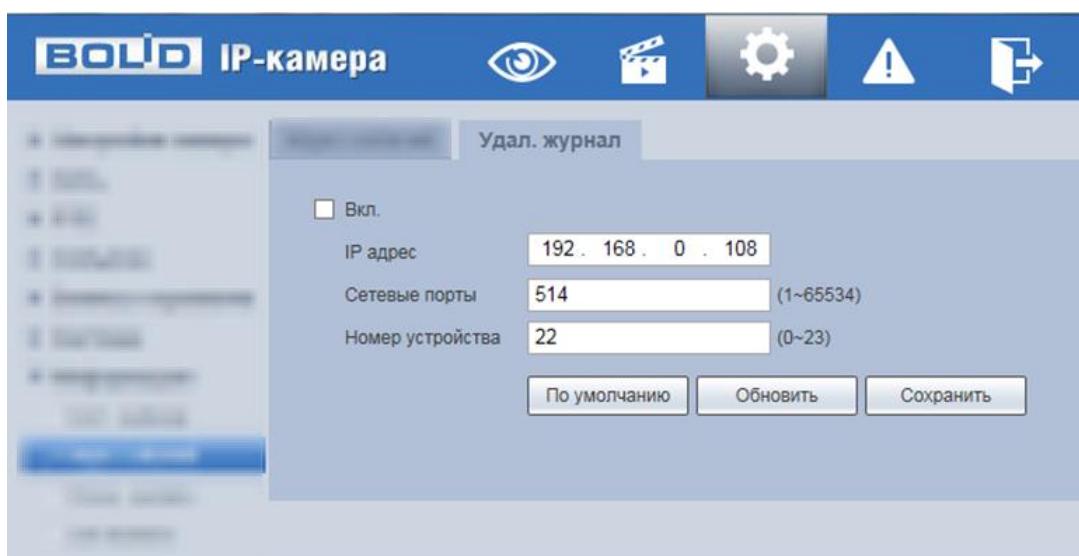
Рисунок 7.127 – Вкладка «Удаленный журнал»
