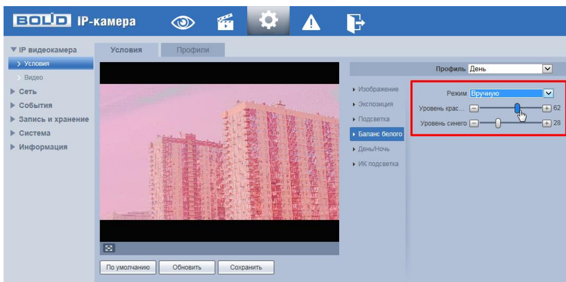
Рисунок 7.33 – Настройка режима баланса белого «Вручную»
