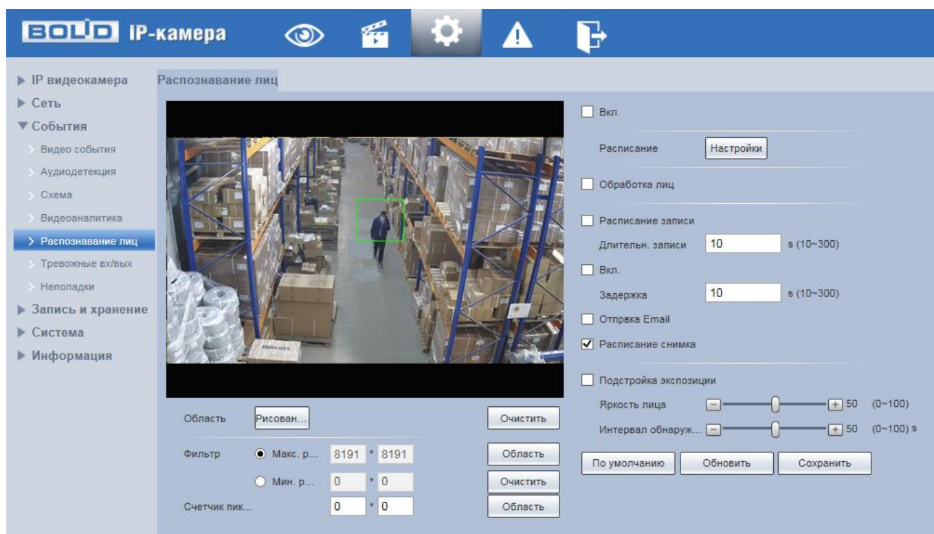
Рисунок 7.84 – Подпункт меню «Распознавание (детекция) лиц»
