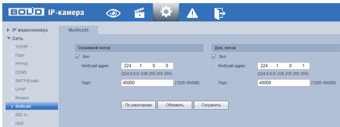
Рисунок 7.62 – Подпункт меню «Multicast»
