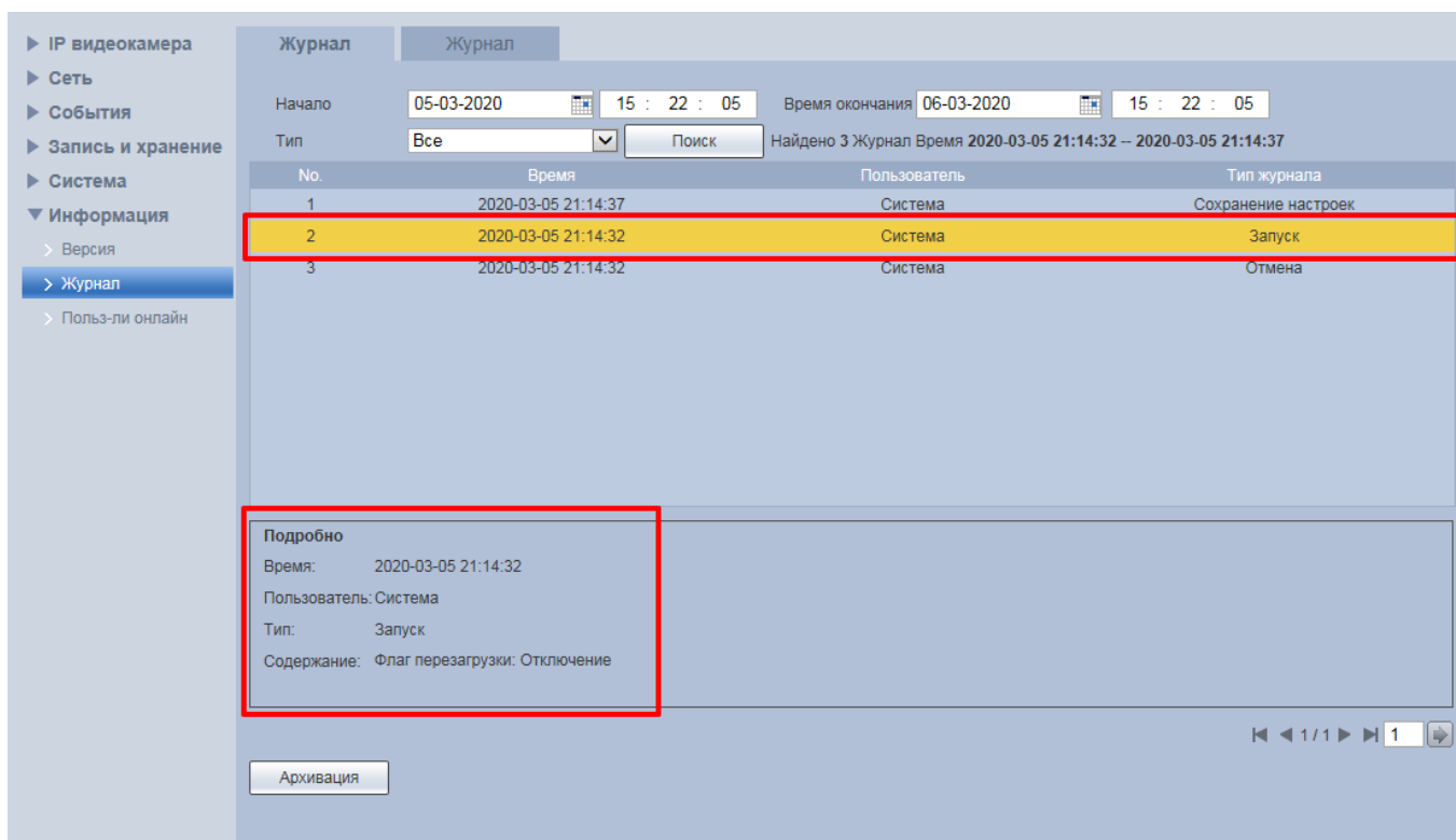
Рисунок 7.126 – Просмотр подробной информации о системном событии
