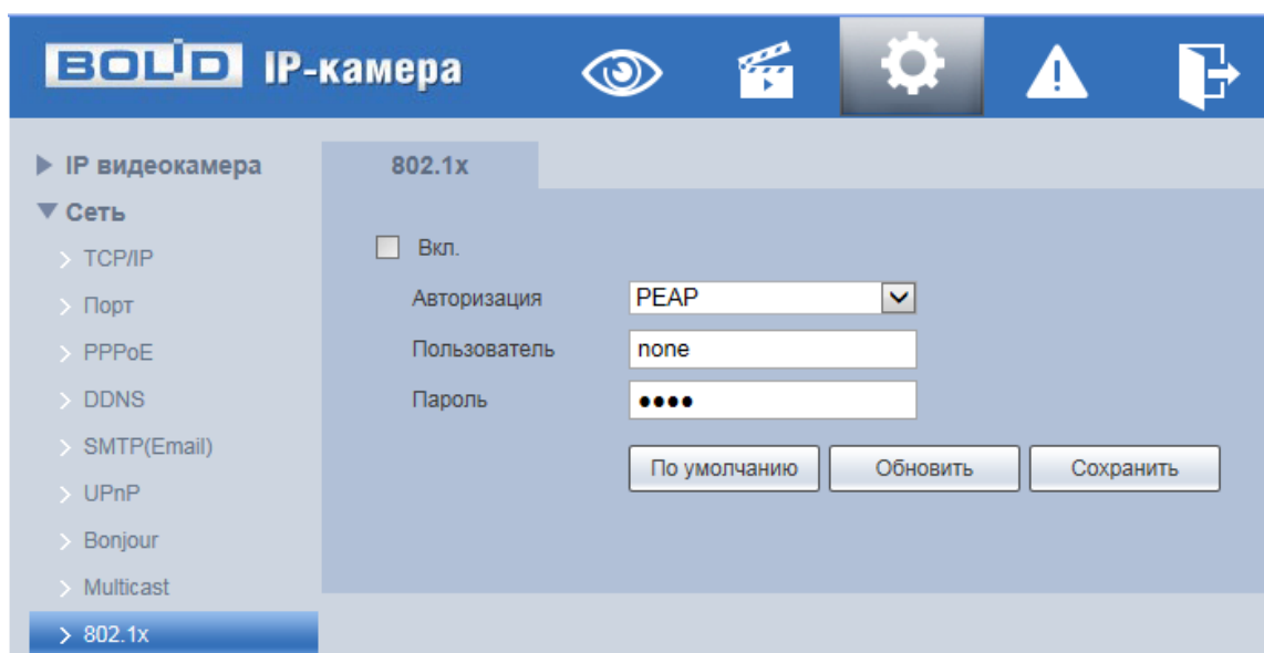
Рисунок 7.63 – Подпункт меню «802.1x»
