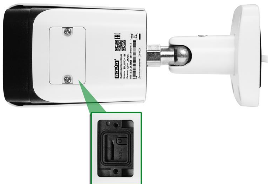
Рисунок 4.2 – Расположение кнопки аппаратного сброса и слота для карты памяти
