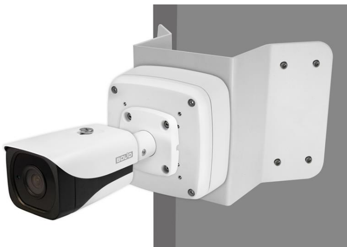
Рисунок 5.7 – Монтаж видеокамеры и монтажной коробки BR-201 на угловом кронштейне BR-102
