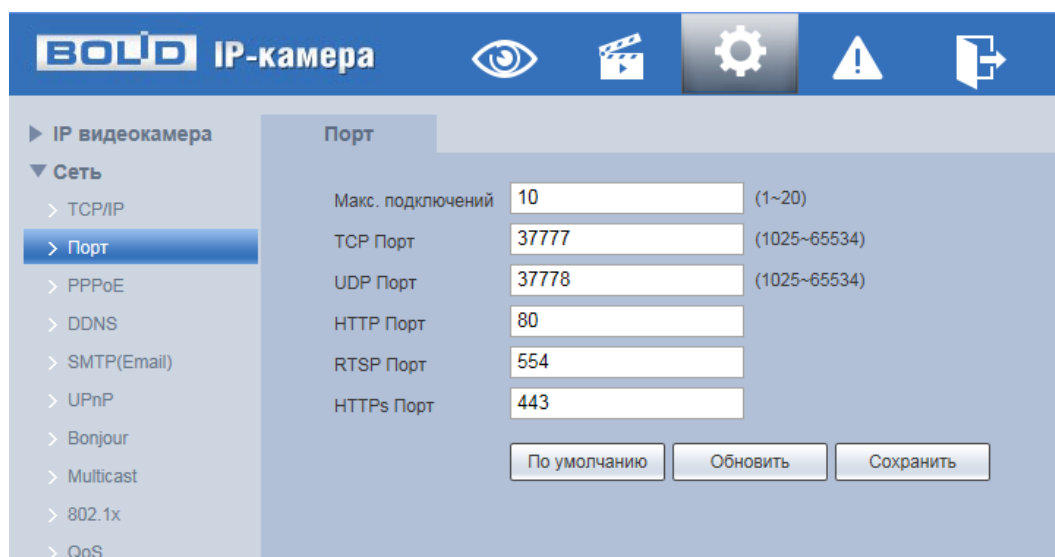
Рисунок 7.53 – Подпункт меню «Порт»
