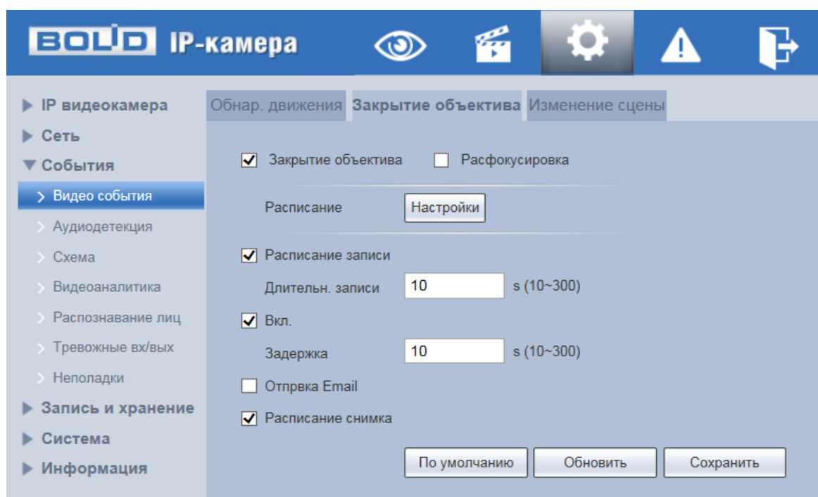
Рисунок 7.75 – Вкладка «Закрытие объектива»
