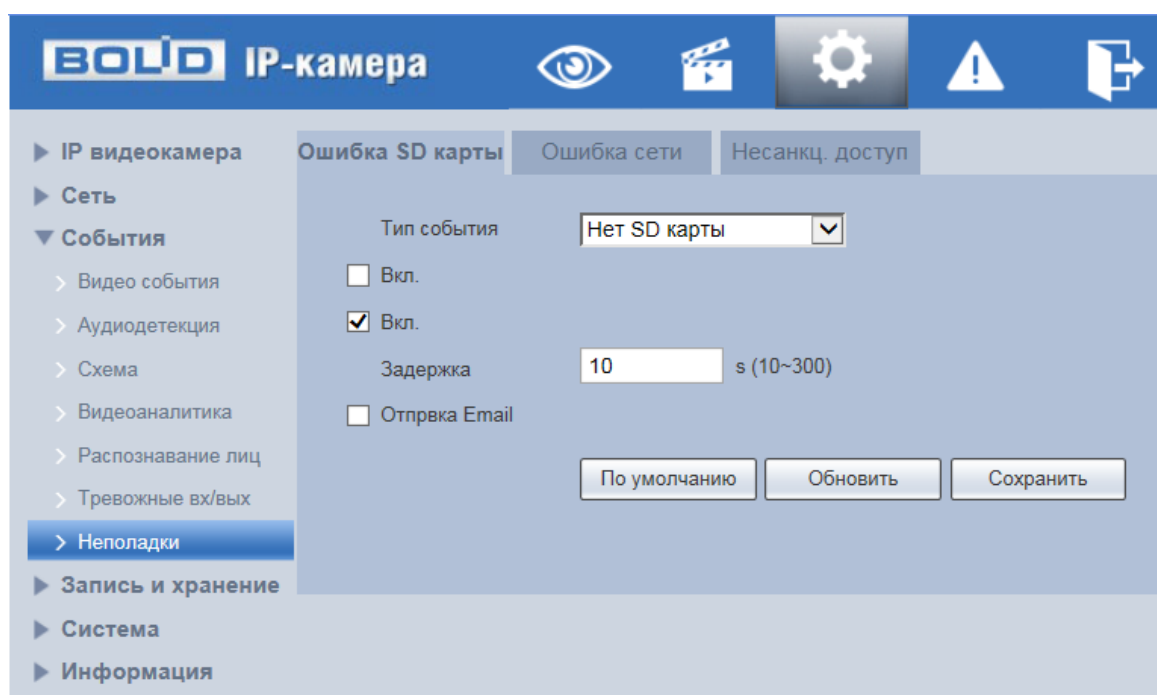
Рисунок 7.87 – Вкладка «Ошибка SD карты»
