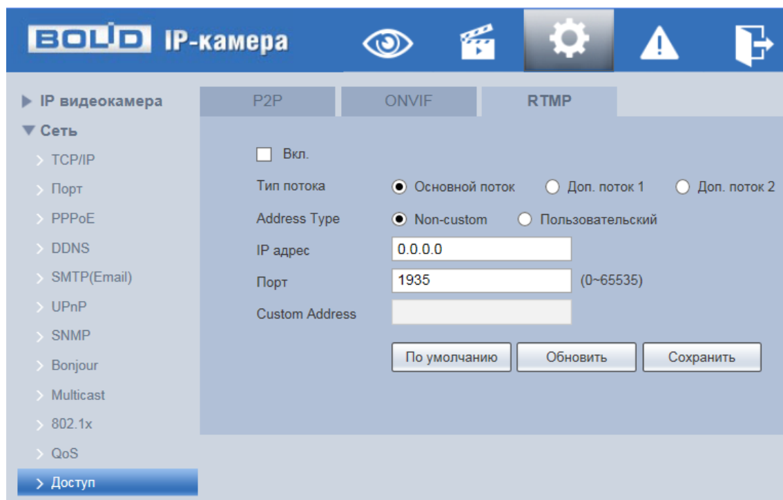
Рисунок 7.68 – Вкладка «RTMP»
