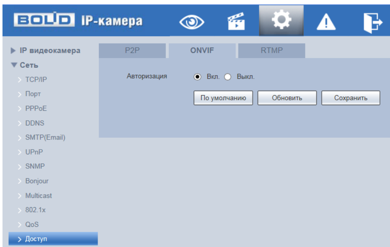
Рисунок 7.67 – Вкладка «ONVIF»
