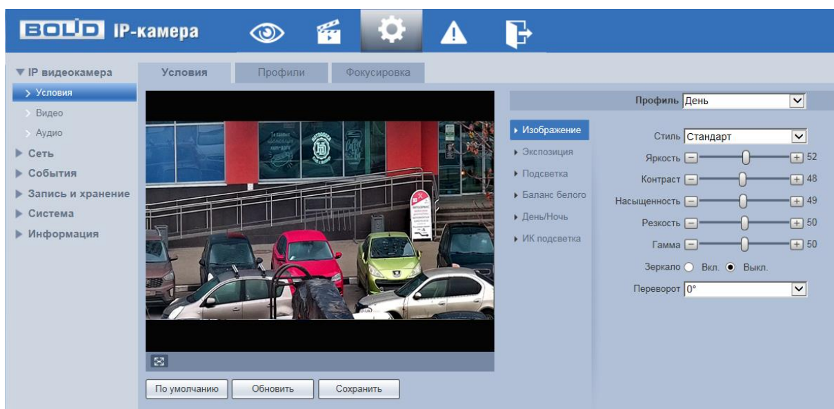
Рисунок 7.27 – Вкладка «Условия»
