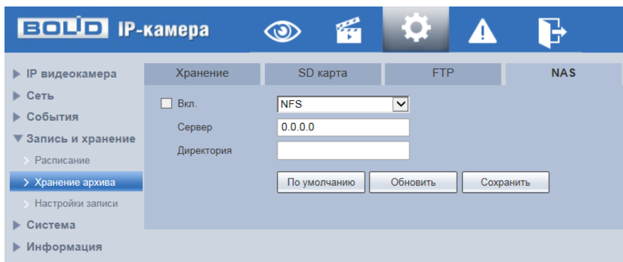
Рисунок 7.102 – Вкладка «NAS»
