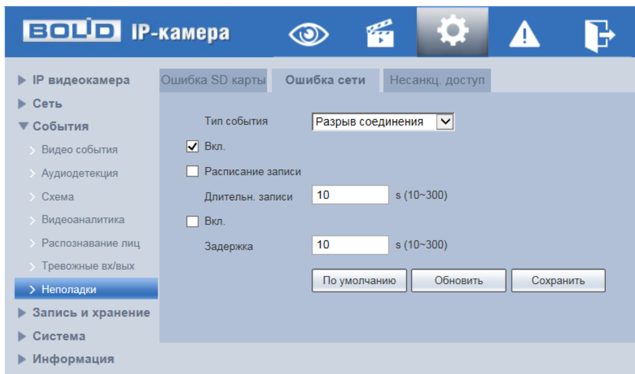
Рисунок 7.88 – Вкладка «Ошибка сети»
