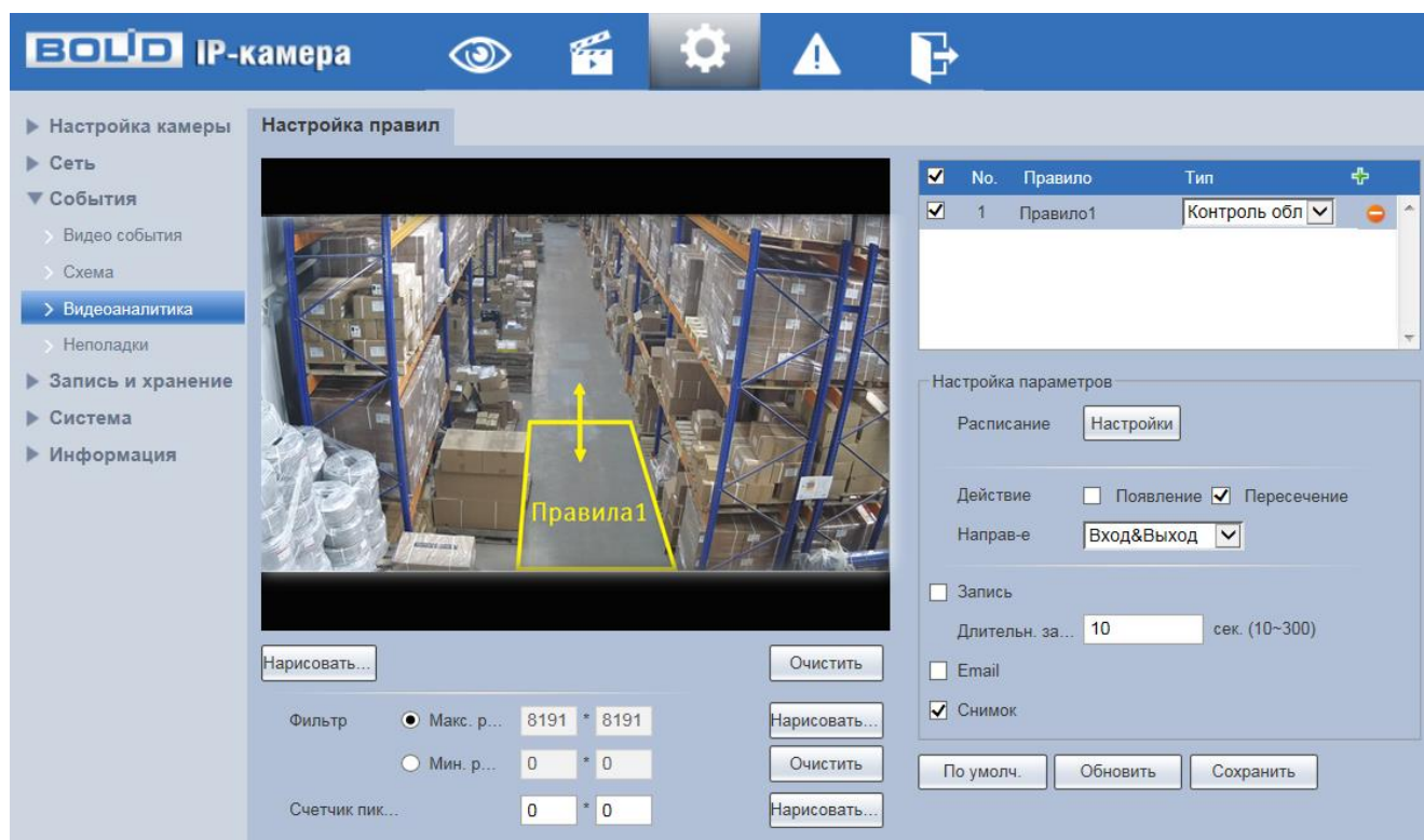
Рисунок 7.83 – Создание правила видеоаналитики «Контроль области»
