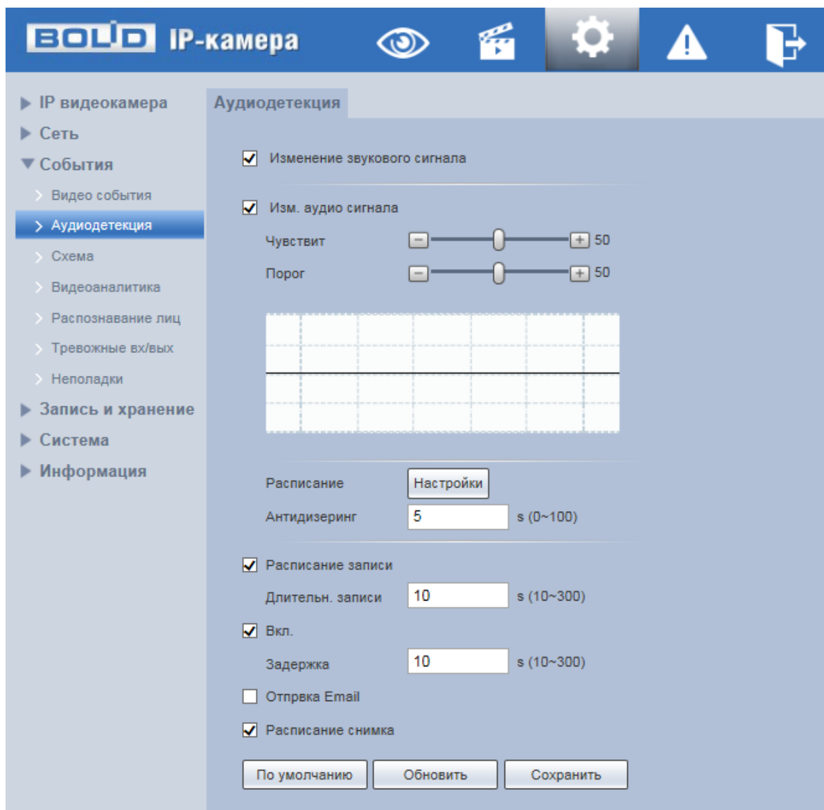
Рисунок 7.79 – Подпункт меню «Аудиодетекция»
