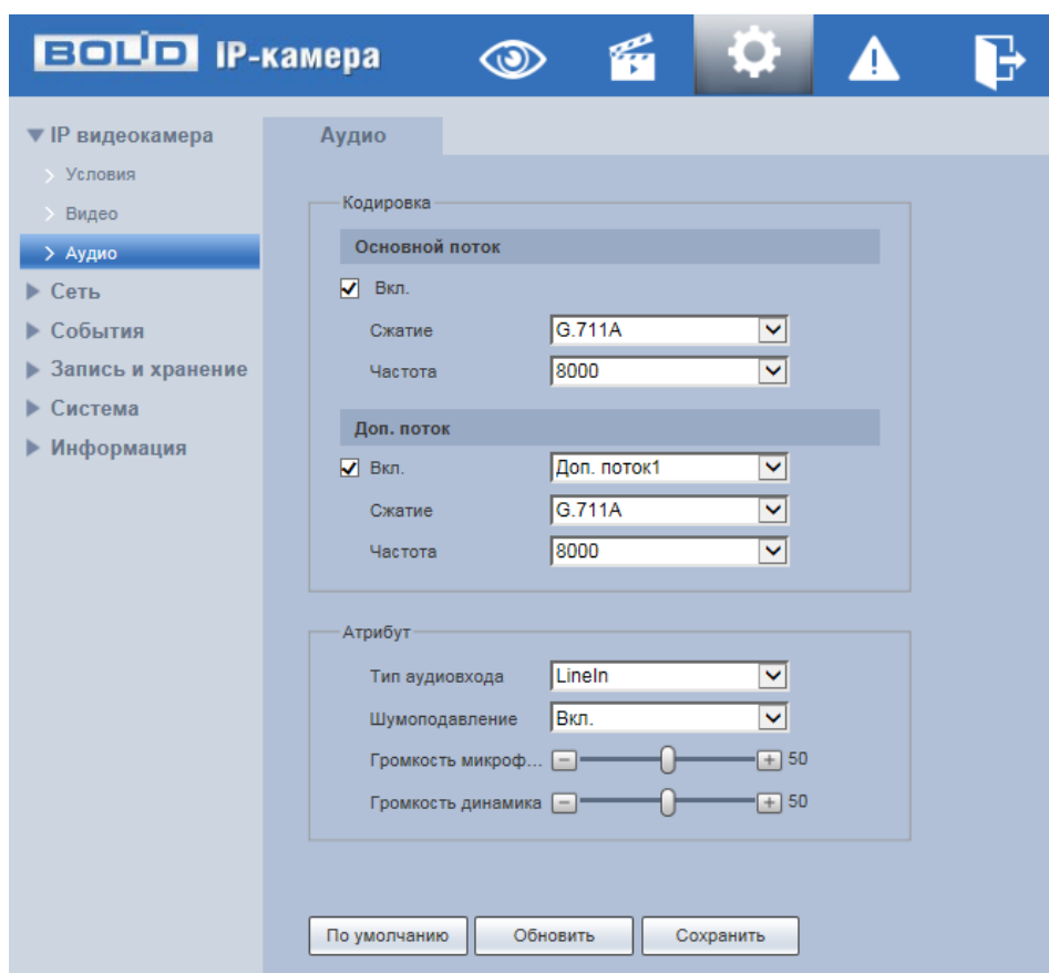
Рисунок 7.49 – Подпункт меню «Аудио»
