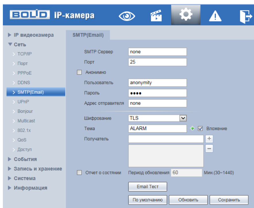
Рисунок 7.57 – Подпункт меню «SMTP»
