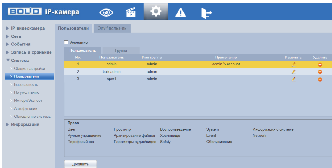
Рисунок 7.110 – Вкладка «Пользователи»
