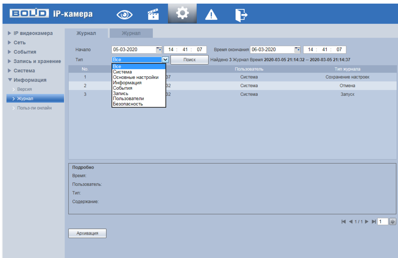
Рисунок 7.125 – Вкладка «Журнал»
