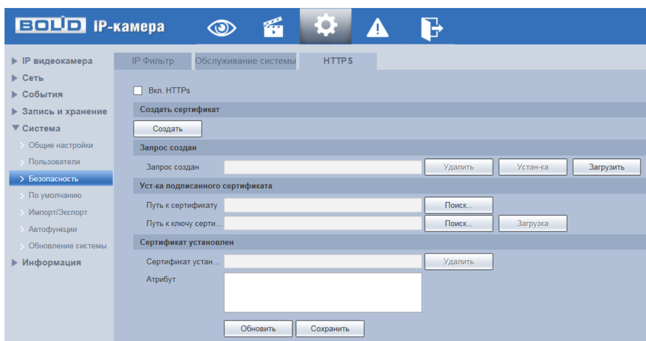
Рисунок 7.116 – Вкладка «HTTPS»
