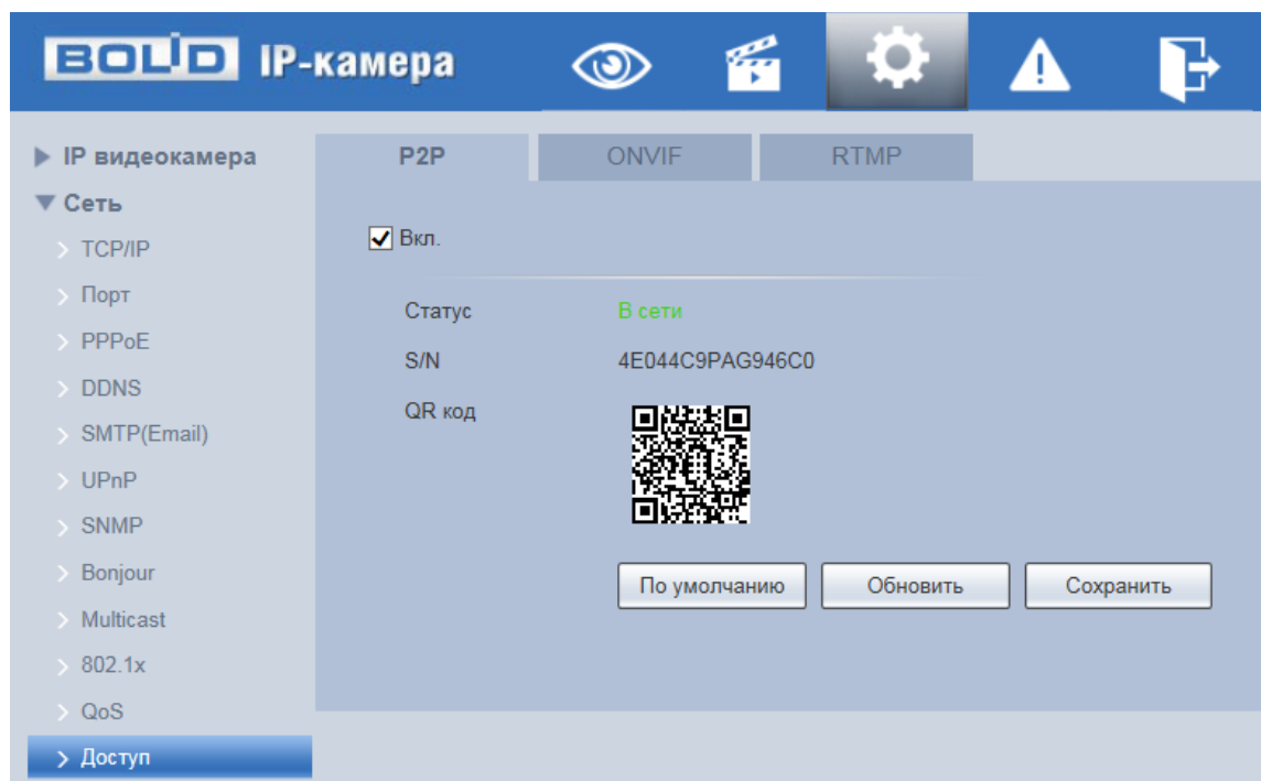
Рисунок 7.66 – Вкладка «P2P»
