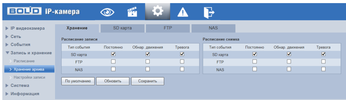
Рисунок 7.99 – Вкладка «Хранение»
