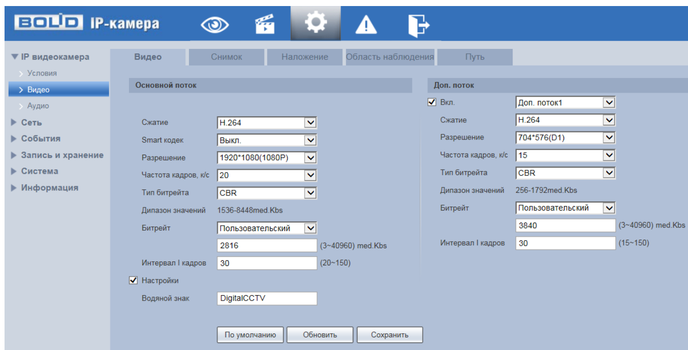
Рисунок 7.38 – Вкладка «Видео»
