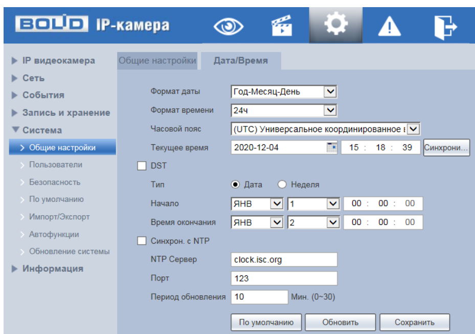
Рисунок 7.108 – Вкладка «Дата/Время»
