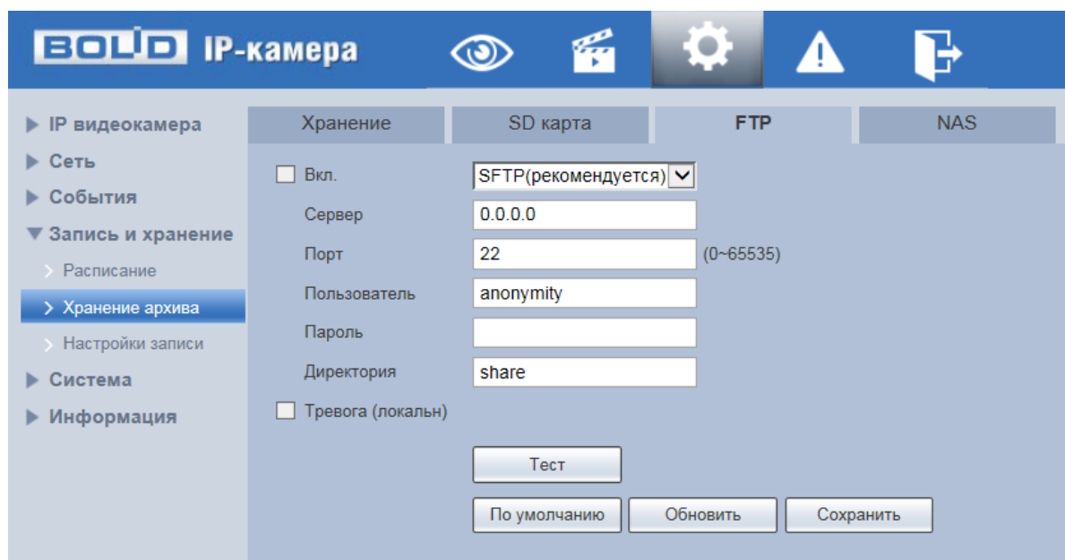
Рисунок 7.101 – Вкладка «FTP»
