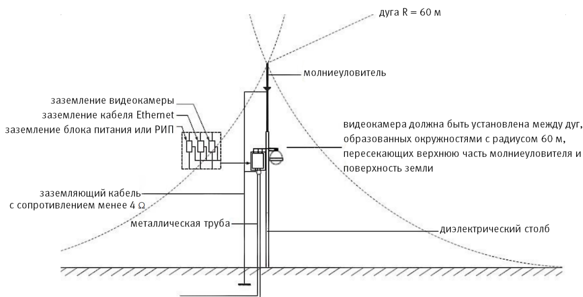
Рисунок 6.13 – Установка молниеотвода
