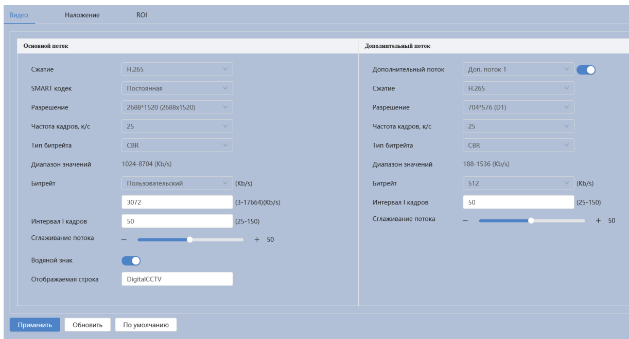
Рисунок 7.70 – Вкладка «Видео»
