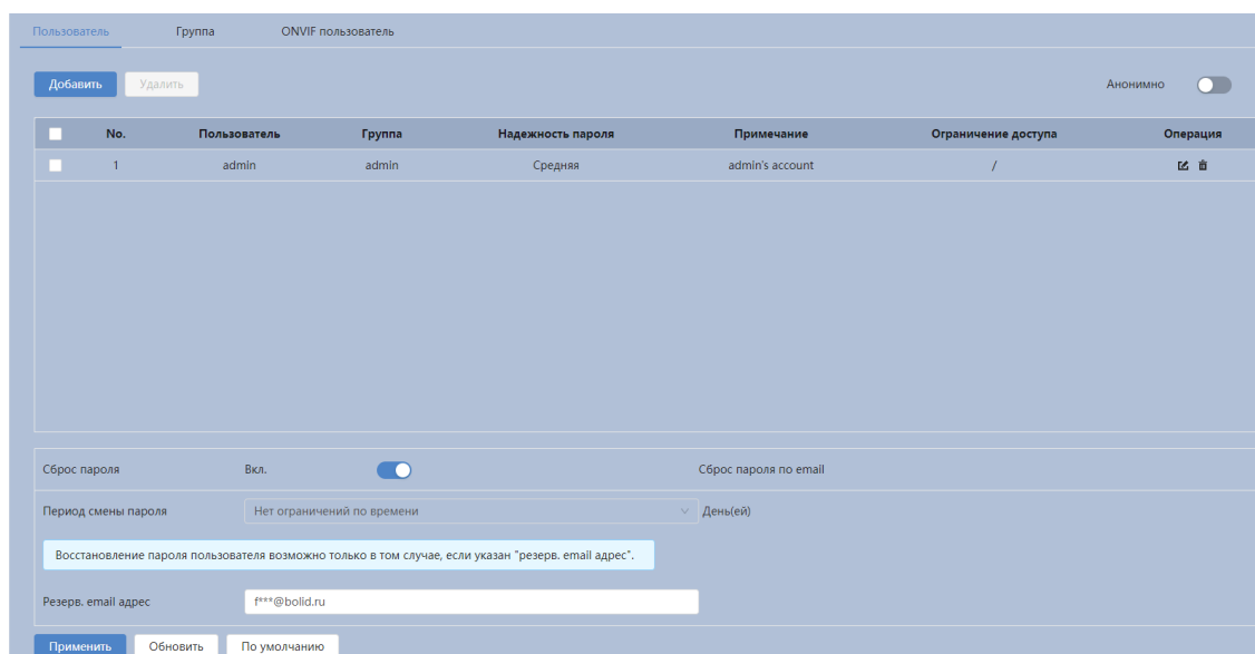
Рисунок 7.105 – Вкладка «Пользователь»
