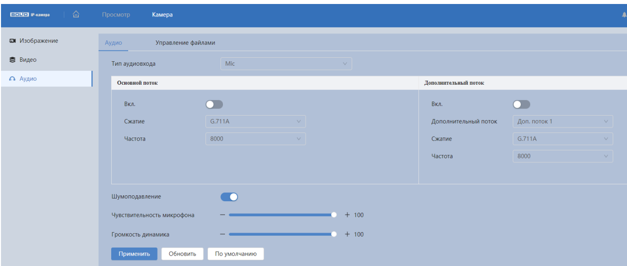
Рисунок 7.82 – Вкладка «Аудио»
