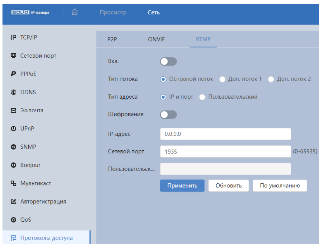
Рисунок 8.21 – Вкладка «RTMP»
