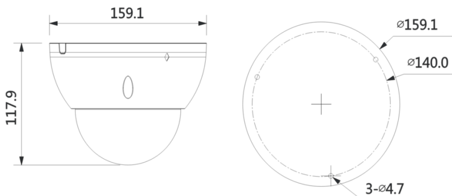
Рисунок 5.1 – Габаритные размеры видеокамеры
