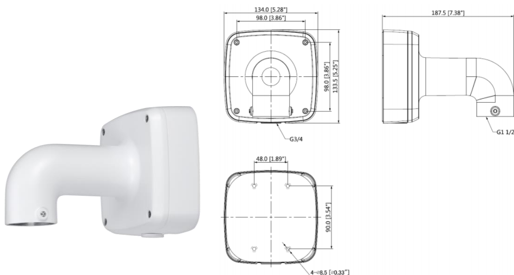
Рисунок 5.12 – Настенный кронштейн BR-107
