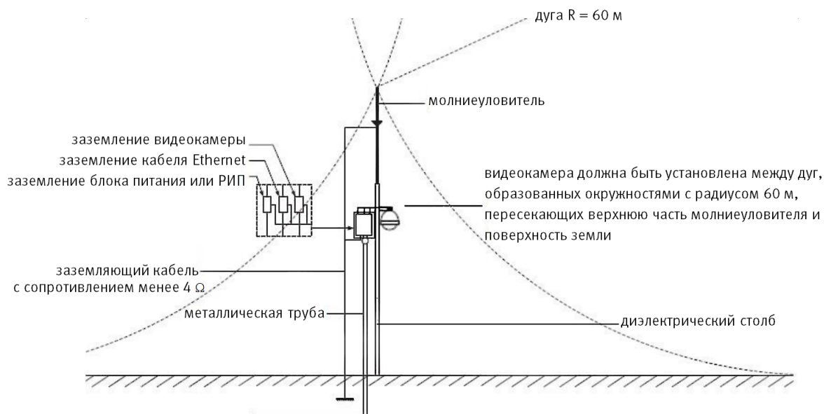
Рисунок 6.13 – Установка молниеотвода
