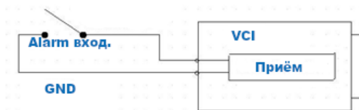
Рисунок 6.12 – Схема подключения тревожного входа
