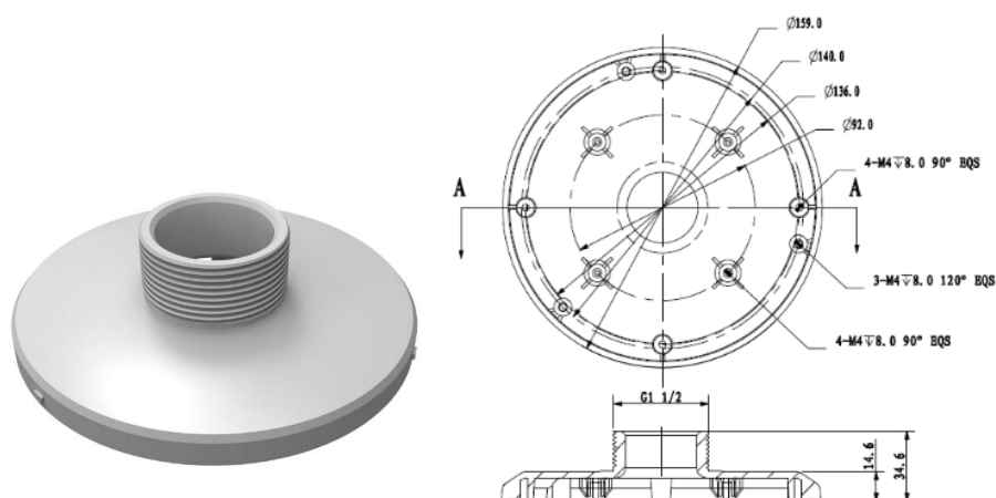
Рисунок 5.5 – Монтажный адаптер BR-303
