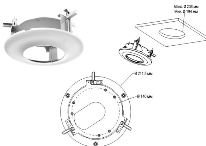
Рисунок 5.9 – Потолочный кронштейн BR-112
