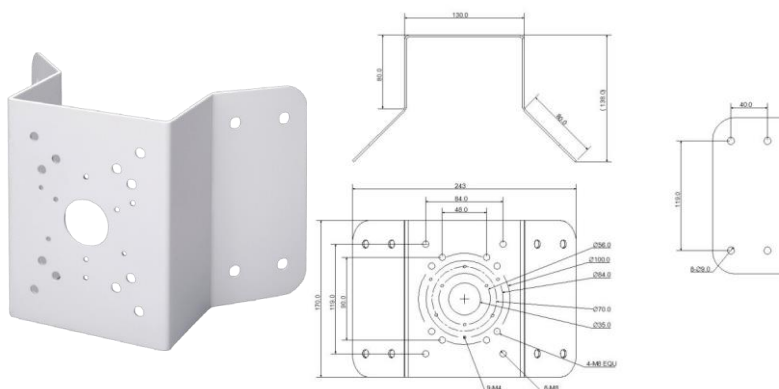
Рисунок 5.14 – Угловой кронштейн BR-102
