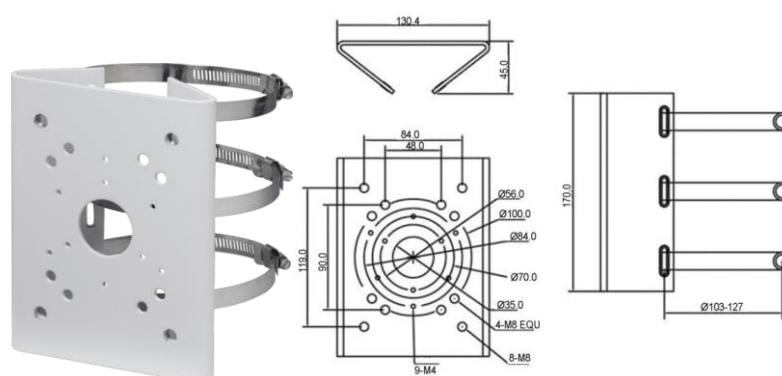
Рисунок 5.17 – Столбовой кронштейн BR-103
