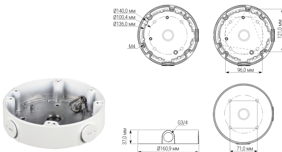
Рисунок 5.7 – Монтажная коробка BR-206
