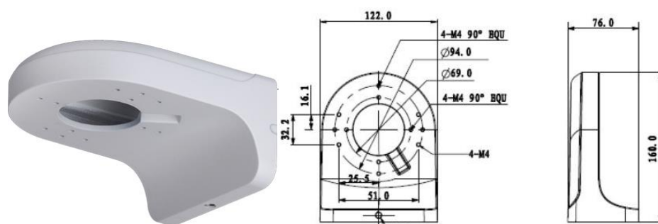
Рисунок 5.8 – Внешний вид и габаритные размеры кронштейна BR-106
