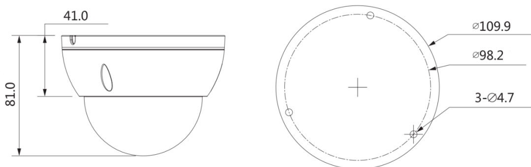
Рисунок 5.1 – Габаритные размеры видеокамеры
