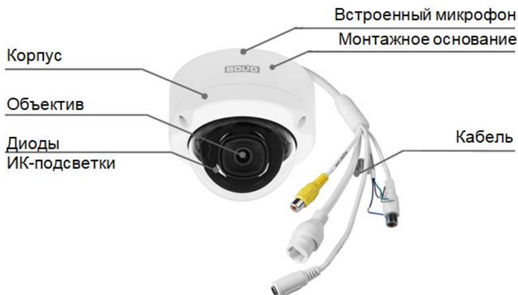
Рисунок 4.1 – Внешний вид и основные элементы видеокамеры
