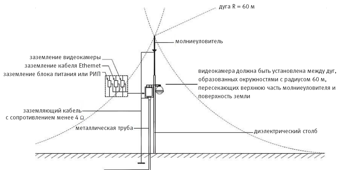
Рисунок 6.13 – Установка молниеотвода
