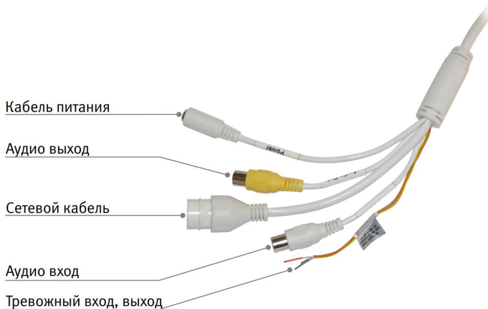
Рисунок 6.1 – Кабель видеоканеры
