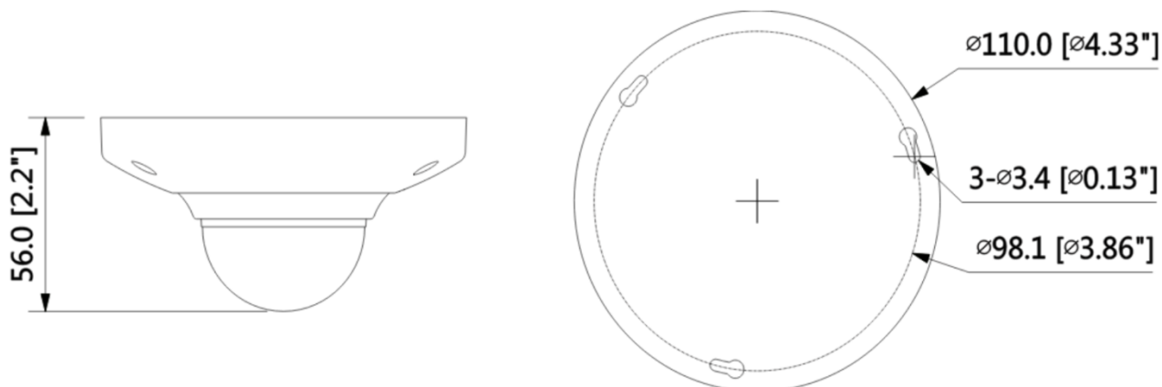
Рисунок 5.1 – Габаритные размеры видеокамеры
