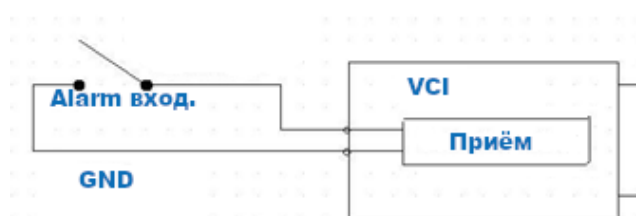
Рисунок 6.12 – Схема подключения тревожного входа
