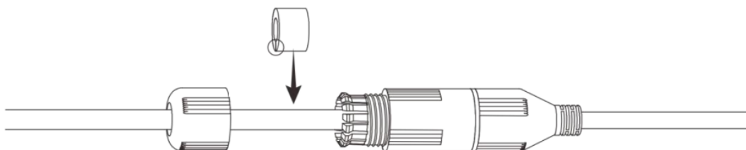
Рисунок 6.9 – Втулка герметичной кабельной муфты
