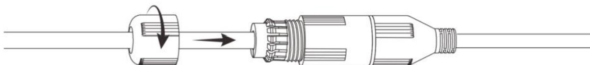
Рисунок 6.10 – Совмещение колпачка с основанием герметичной кабельной муфты
