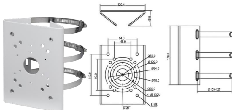
Рисунок 5.17 – Столбовой кронштейн BR-103
