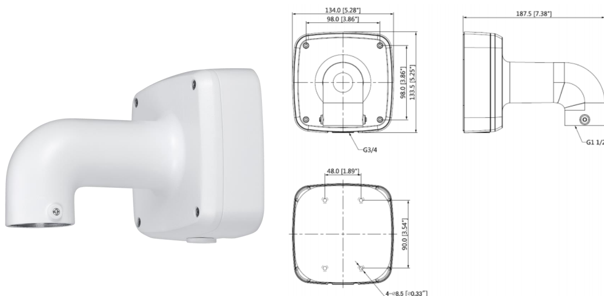
Рисунок 5.12 – Настенный кронштейн BR-107
