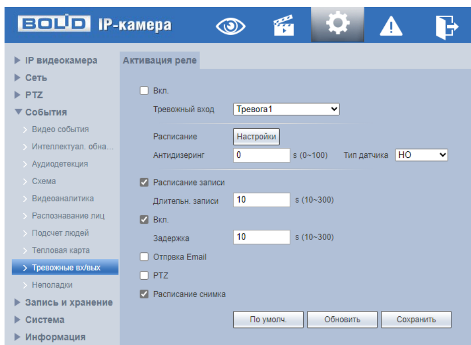
Рисунок 9.103 – Подпункт меню «Тревожные входы/выходы»
