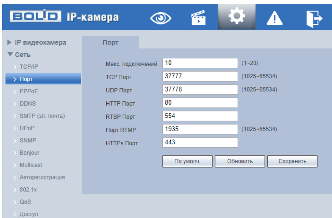
Рисунок 9.52 – Подпункт меню «Порт»
