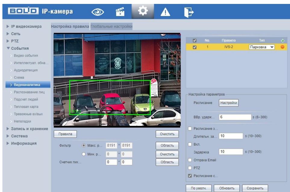
Рисунок 9.87 – Создание правила видеоаналитики «Парковка»
