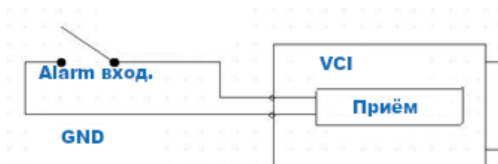
Рисунок 6.5 – Схема подключения тревожного входа
