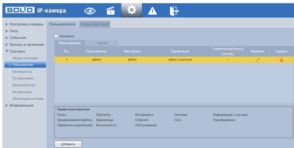
Рисунок 7.100 – Вкладка «Пользователи»
