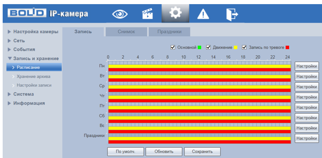
Рисунок 7.83 – Вкладка «Запись»
