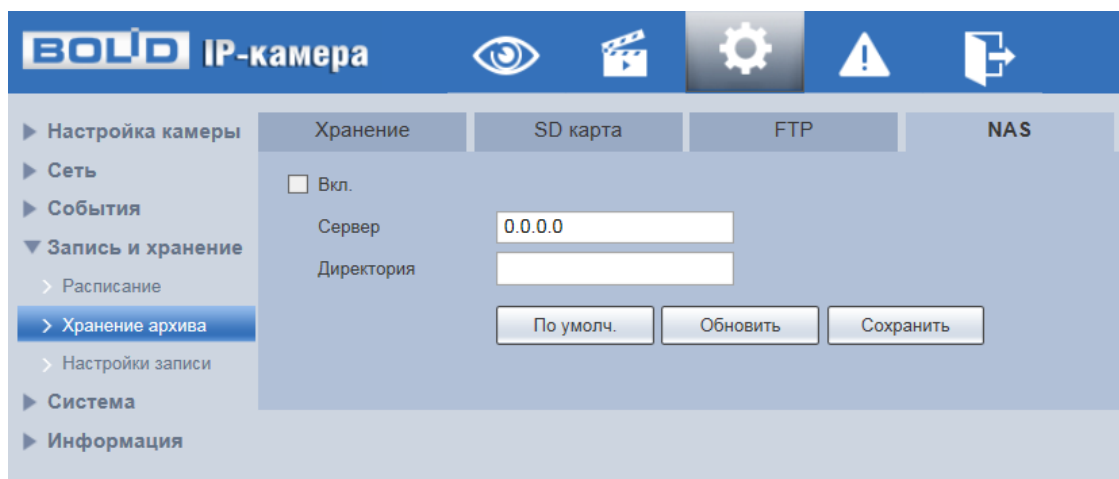
Рисунок 7.92 – Вкладка «NAS»
