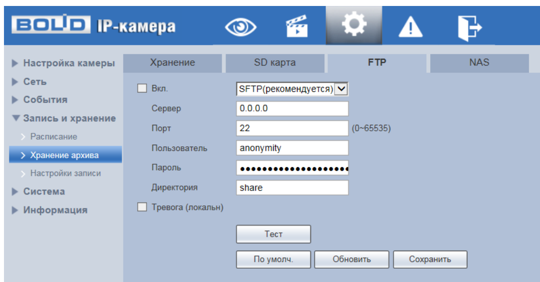
Рисунок 7.91 – Вкладка «FTP»
