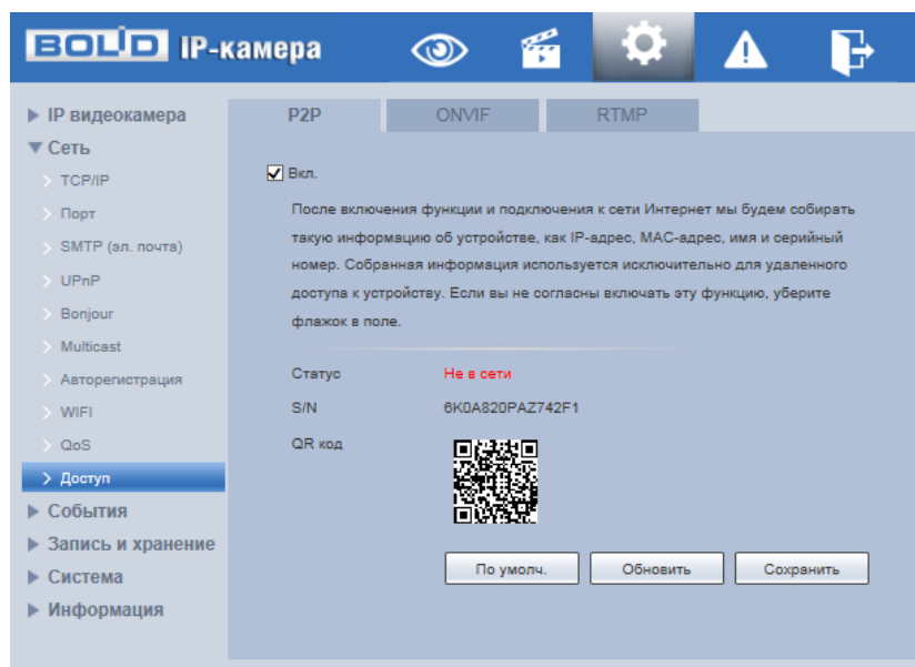
Рисунок 7.62 – Вкладка «P2P»
