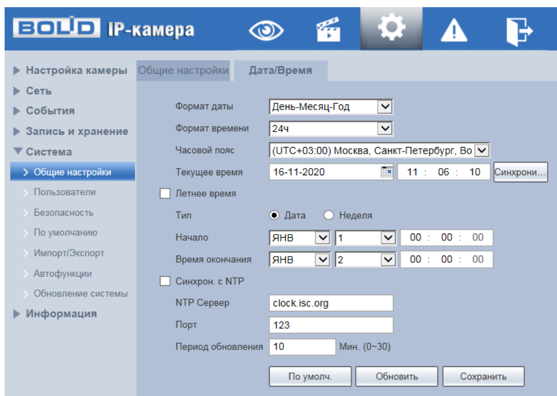
Рисунок 7.98 – Вкладка «Дата/Время»
