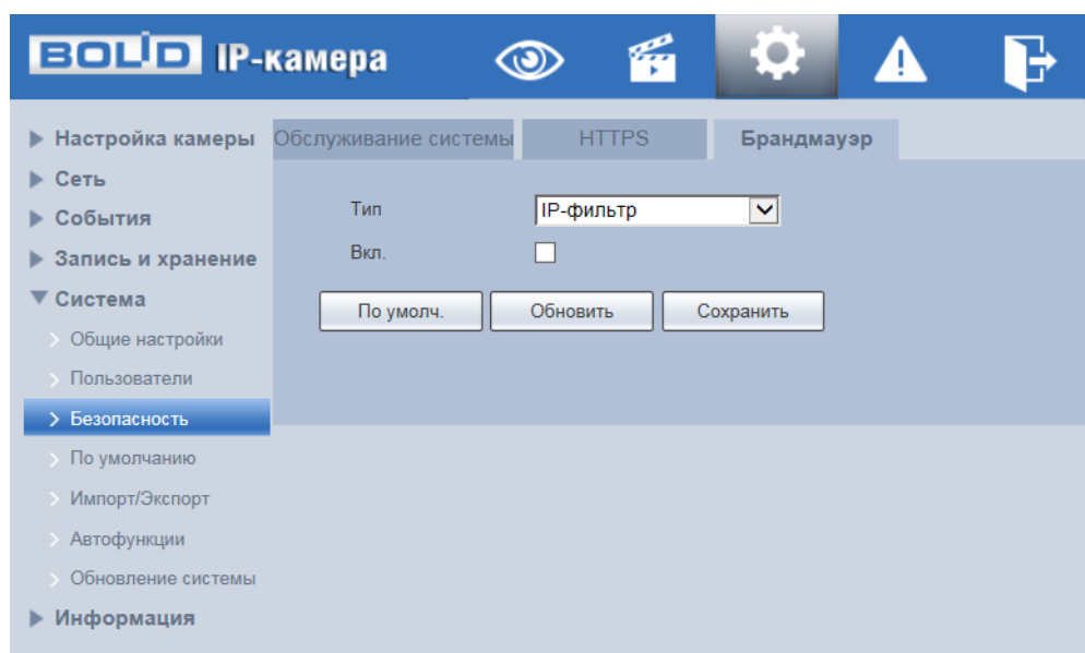
Рисунок 7.106 – Вкладка «Брандмауэр»
