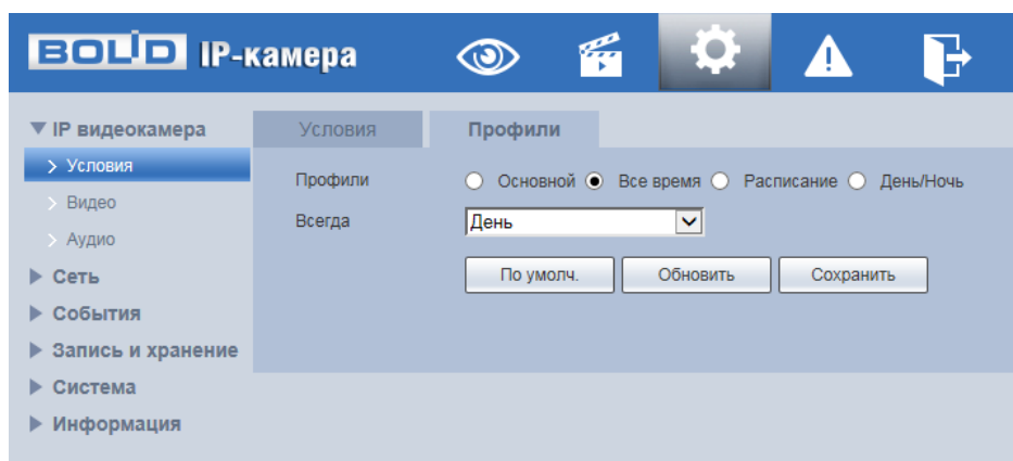
Рисунок 7.36 – Вкладка «Профили»
