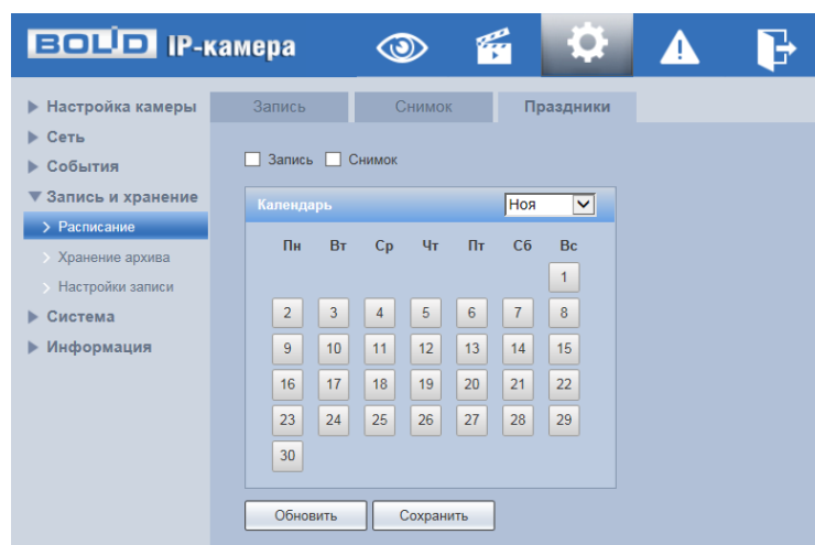
Рисунок 7.87 – Вкладка «Праздники»
