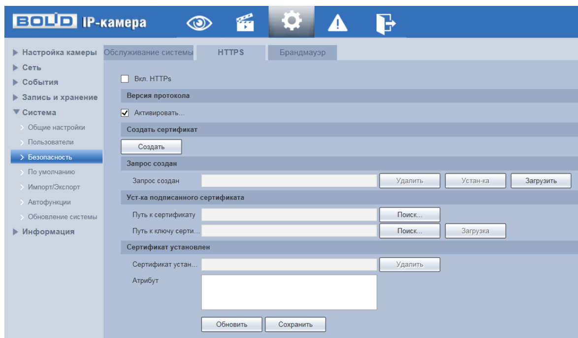
Рисунок 7.104 – Вкладка «HTTPS»
