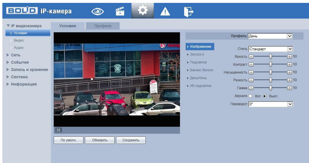
Рисунок 7.27 – Вкладка «Условия»
