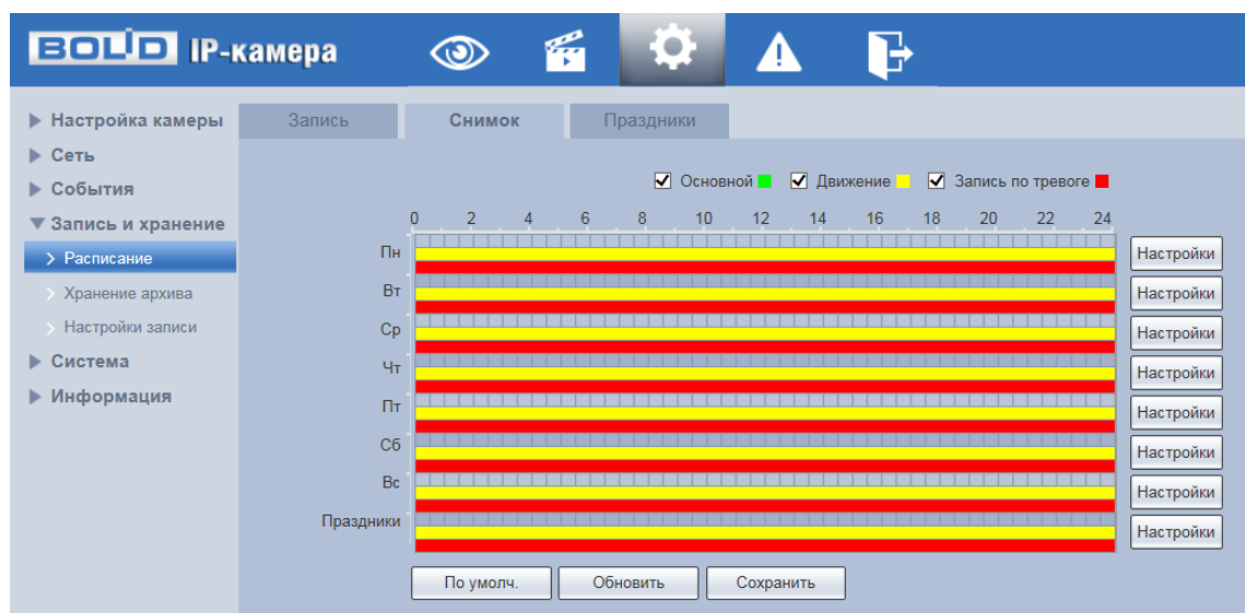
Рисунок 7.85 – Вкладка «Снимок»
