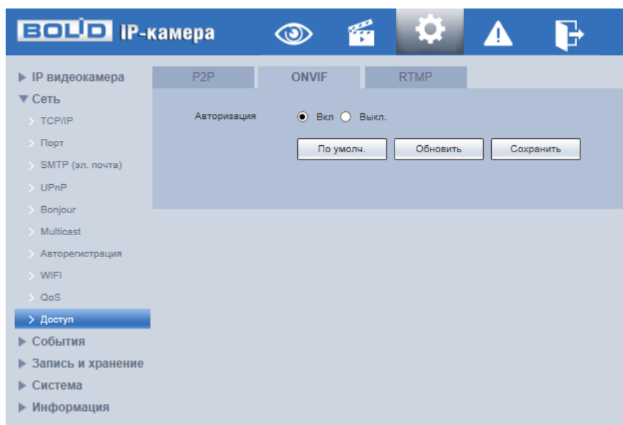
Рисунок 7.63 – Вкладка «ONVIF»
