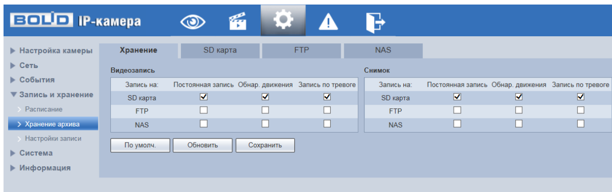
Рисунок 7.89 – Вкладка «Хранение»
