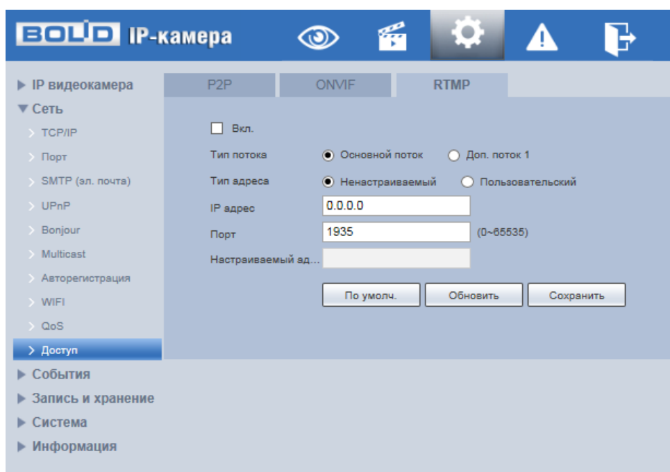
Рисунок 7.64 – Вкладка «RTMP»
