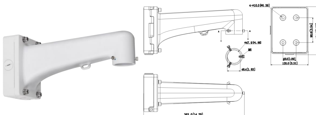
Рисунок 5.10 – Настенный кронштейн BR-110
