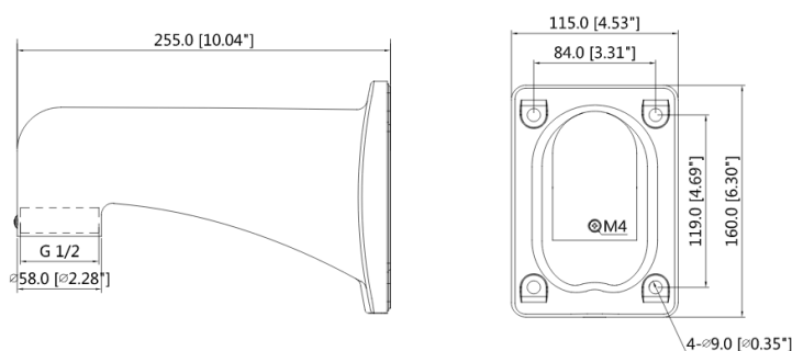
Рисунок 5.6 – Габаритные размеры настенного кронштейна
