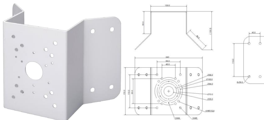
Рисунок 5.12 – Угловой кронштейн BR-102
