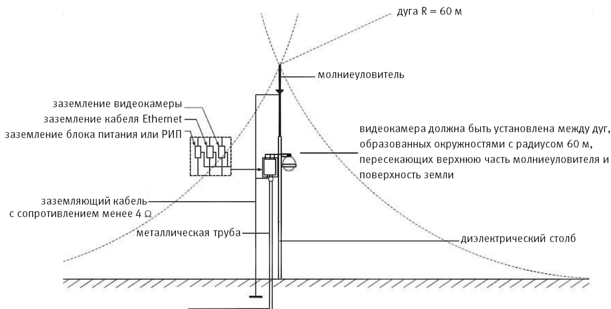
Рисунок 6.13 – Установка молниеотвода
