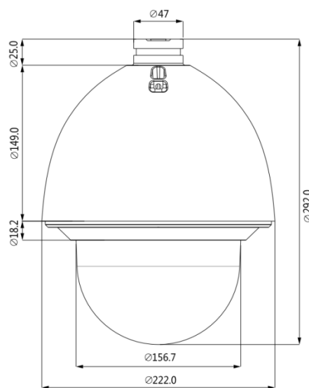
Рисунок 5.1 – Габаритные размеры видеокамеры (мм)
