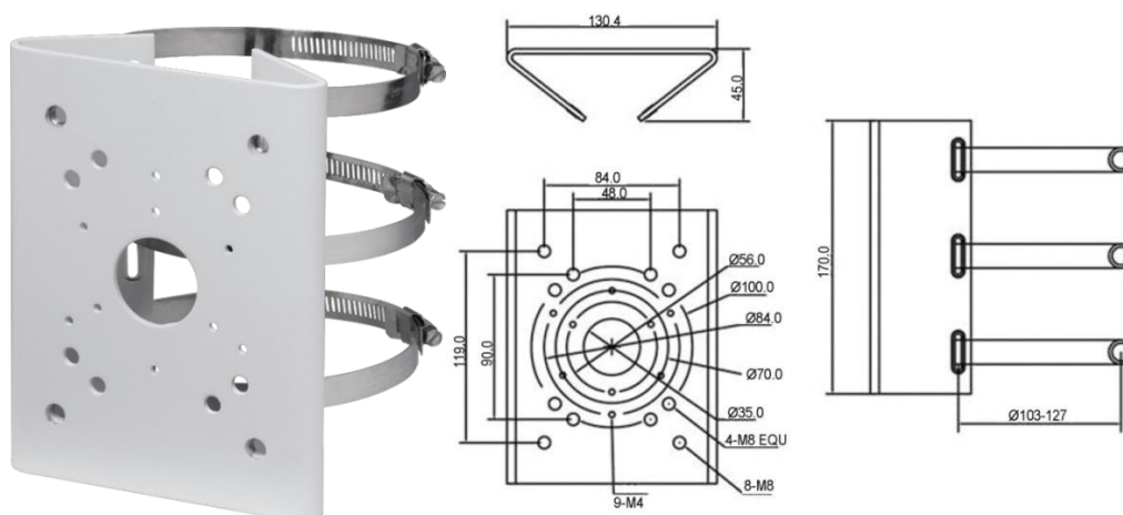
Рисунок 5.15 – Столбовой кронштейн BR-103
