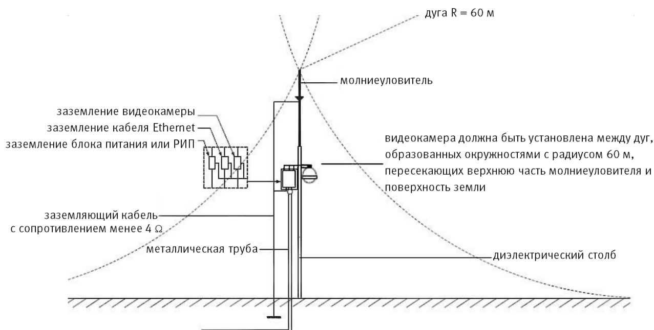
Рисунок 6.13 – Установка молниеотвода
