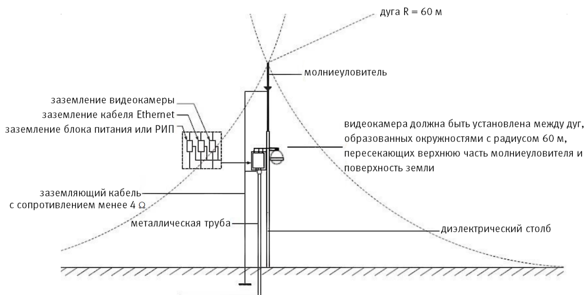
Рисунок 6.13 – Установка молниеотвода
