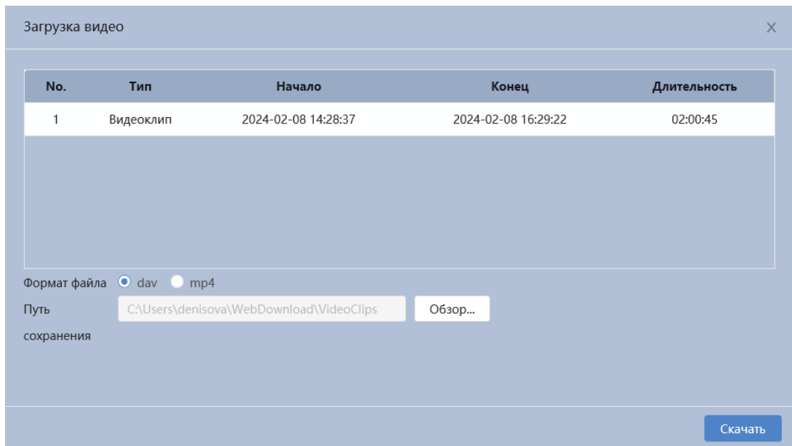
Рисунок 7.130 – Загрузка видео
