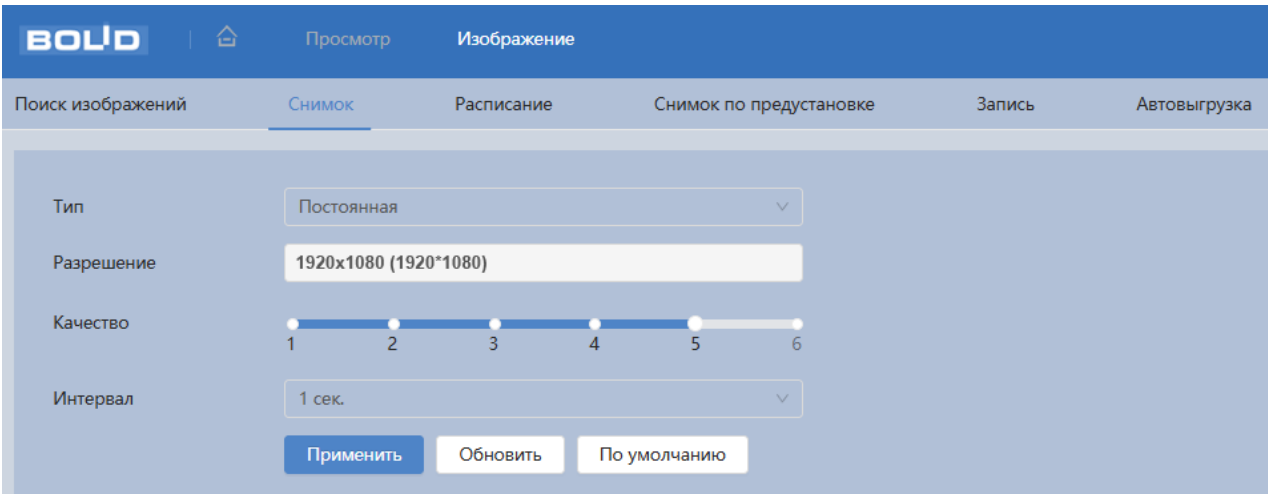
Рисунок 7.137 – Вкладка «Снимок»
