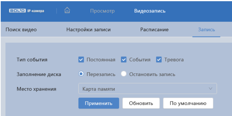
Рисунок 7.134 – Вкладка «Запись»
