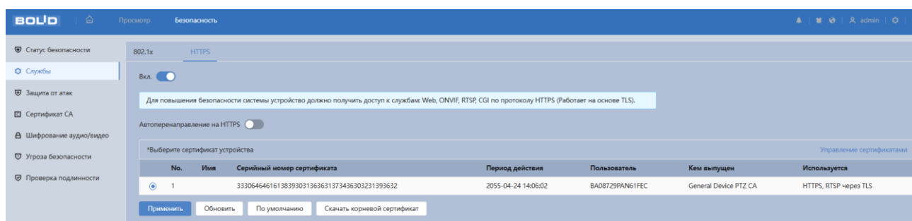
Рисунок 7.149 – Вкладка «HTTPS»
