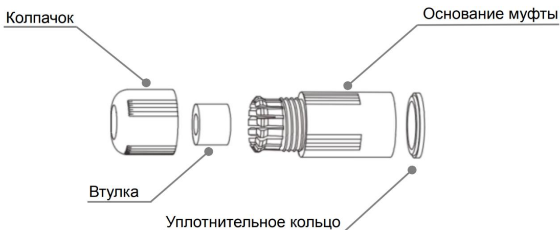
Рисунок 6.5 – Элементы герметичной кабельной муфты
