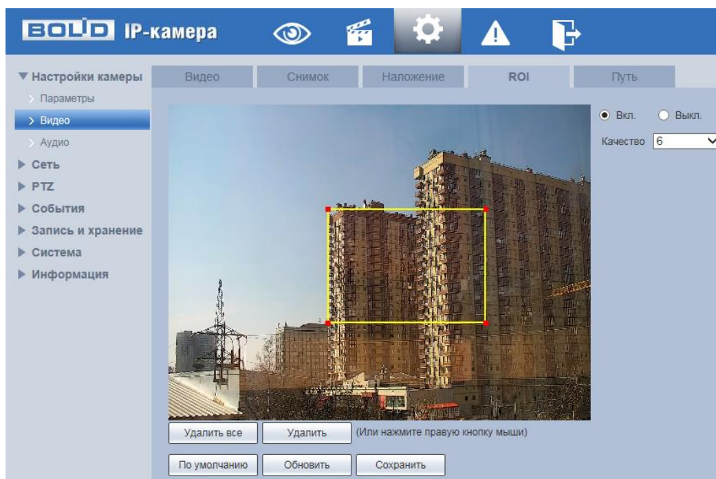
Рисунок 7.48 – Вкладка «ROI»
