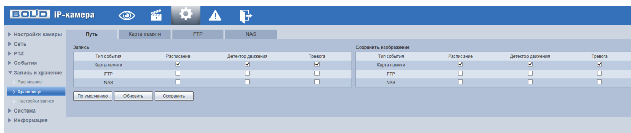
Рисунок 7.138 – Вкладка «Путь»
